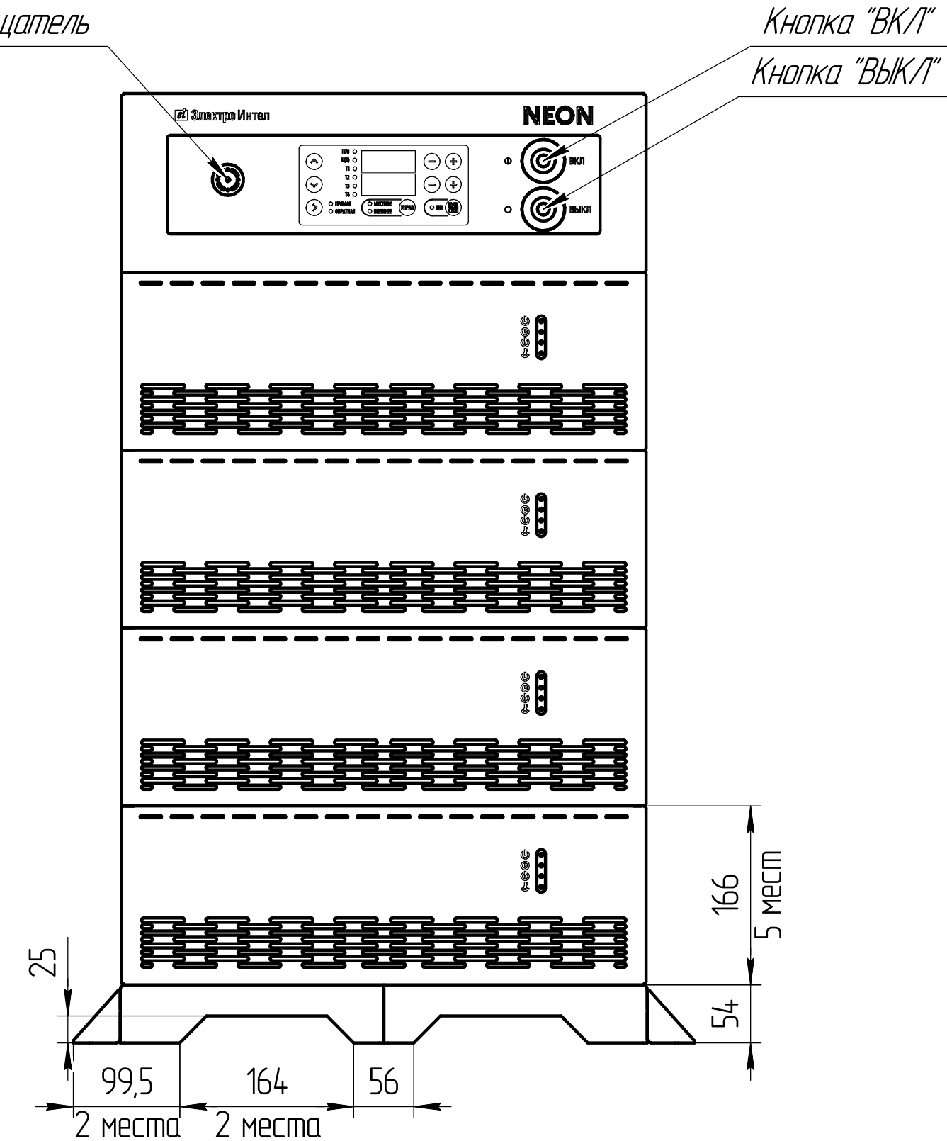
Вид спереди
