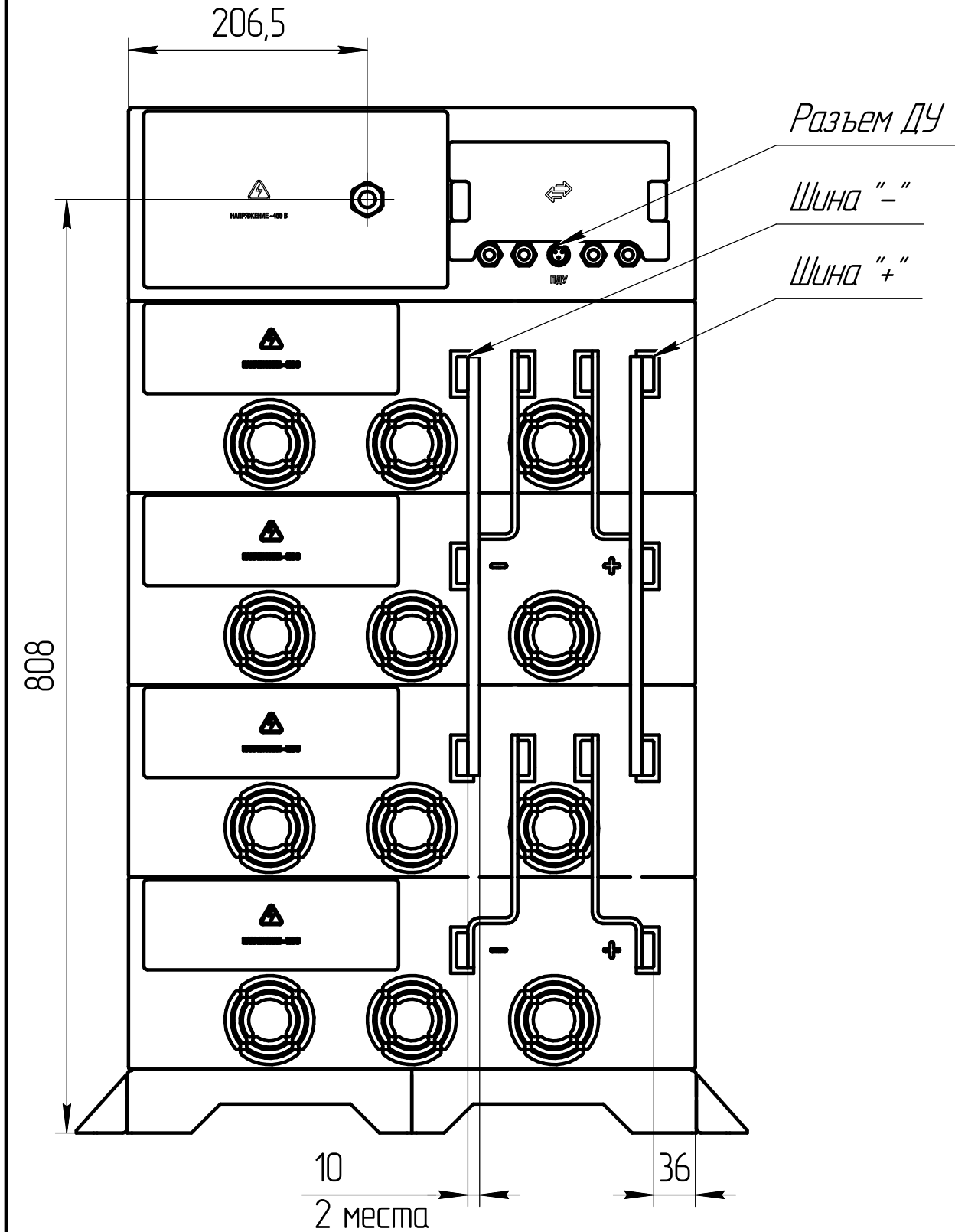
Вид сзади
