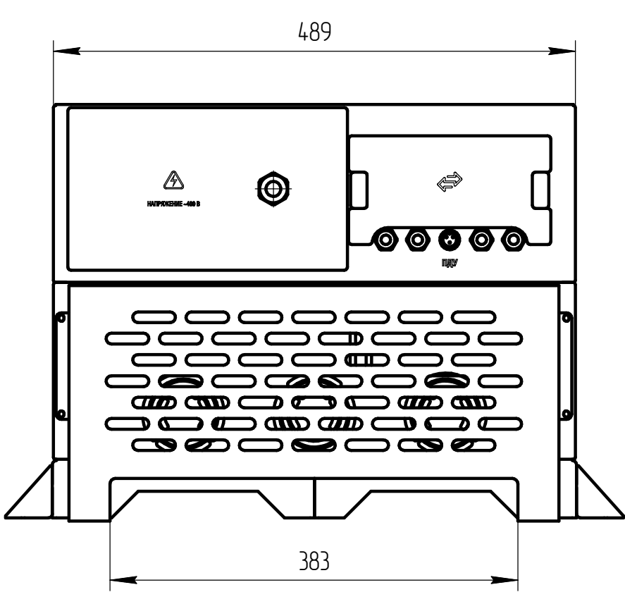
Вид сзади
