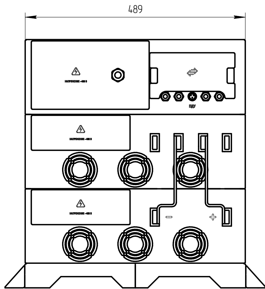
Вид сзади
