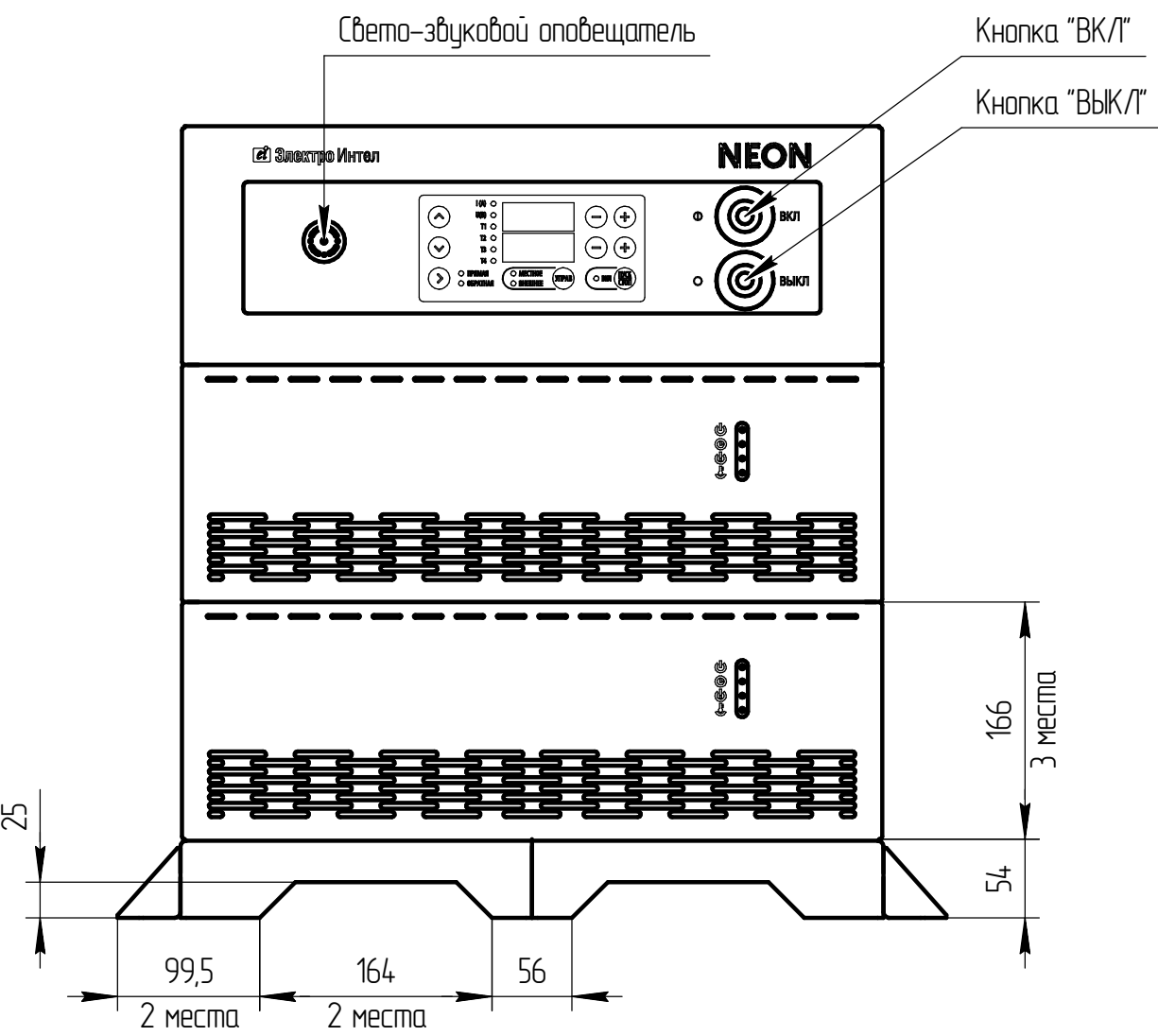
Вид спереди
