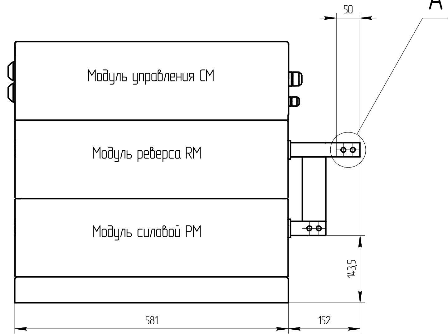
Вид сверху
