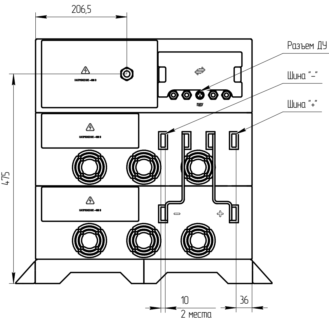
Вид сзади
