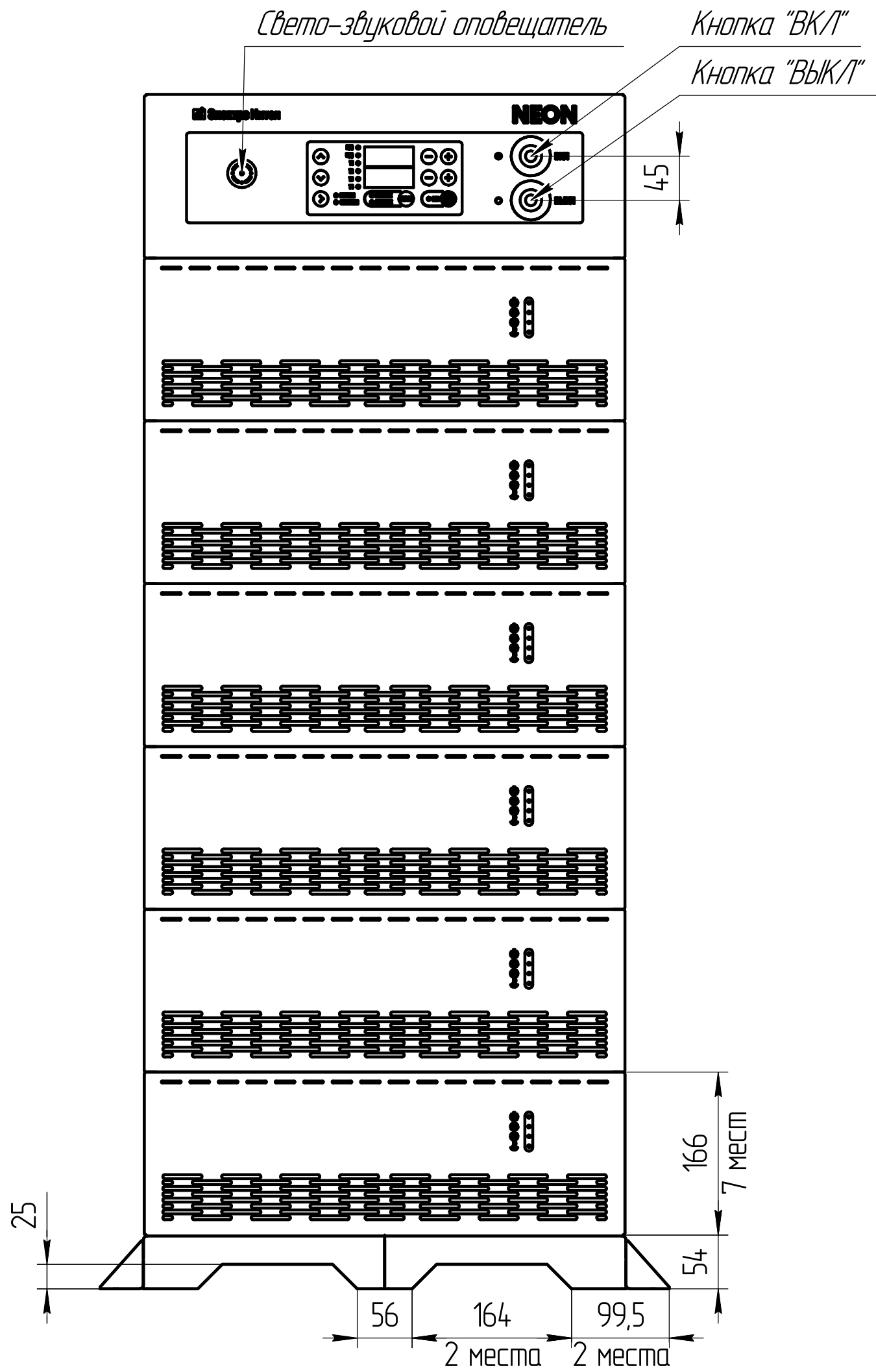
Вид спереди
