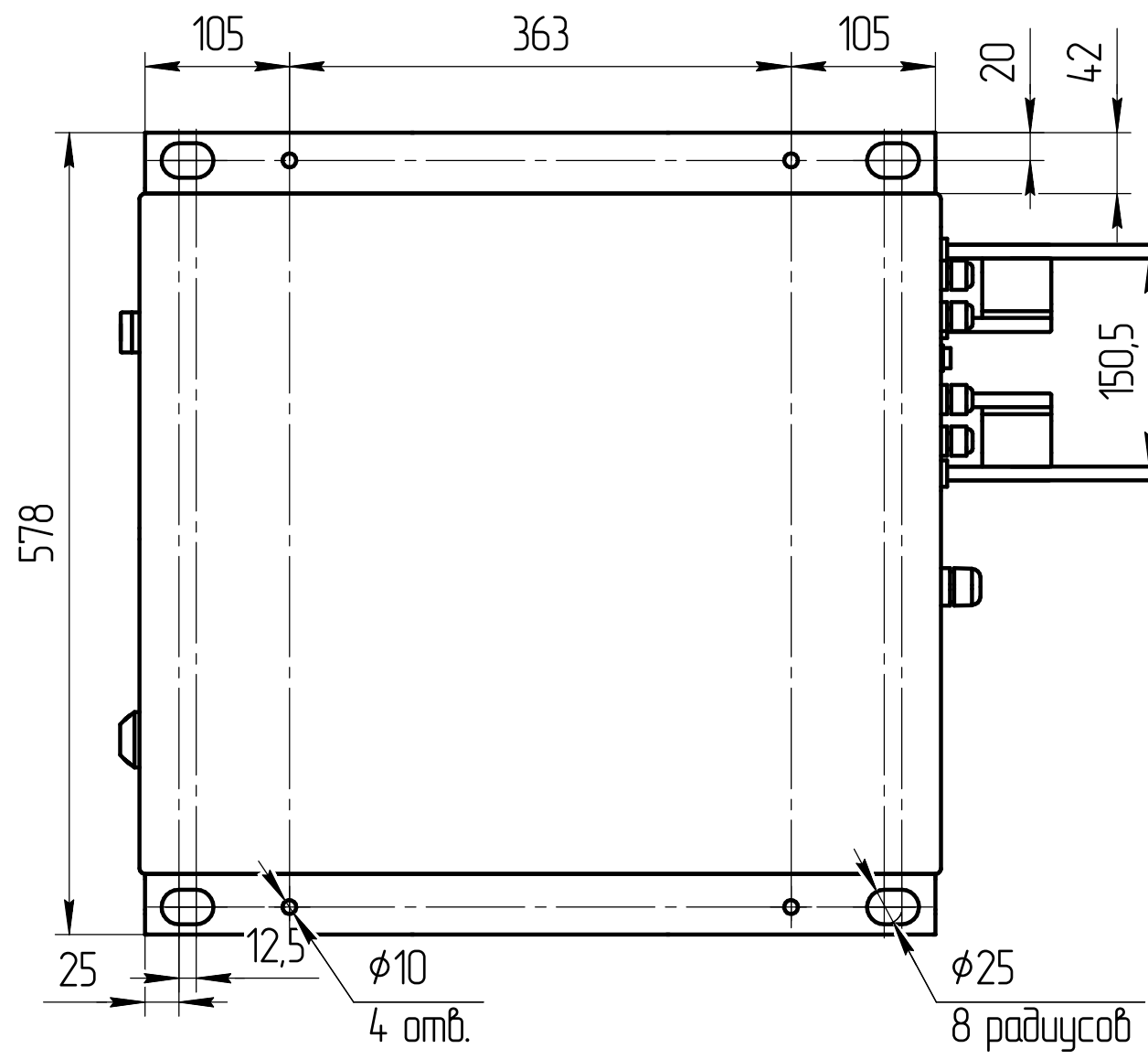
Вид сверху
