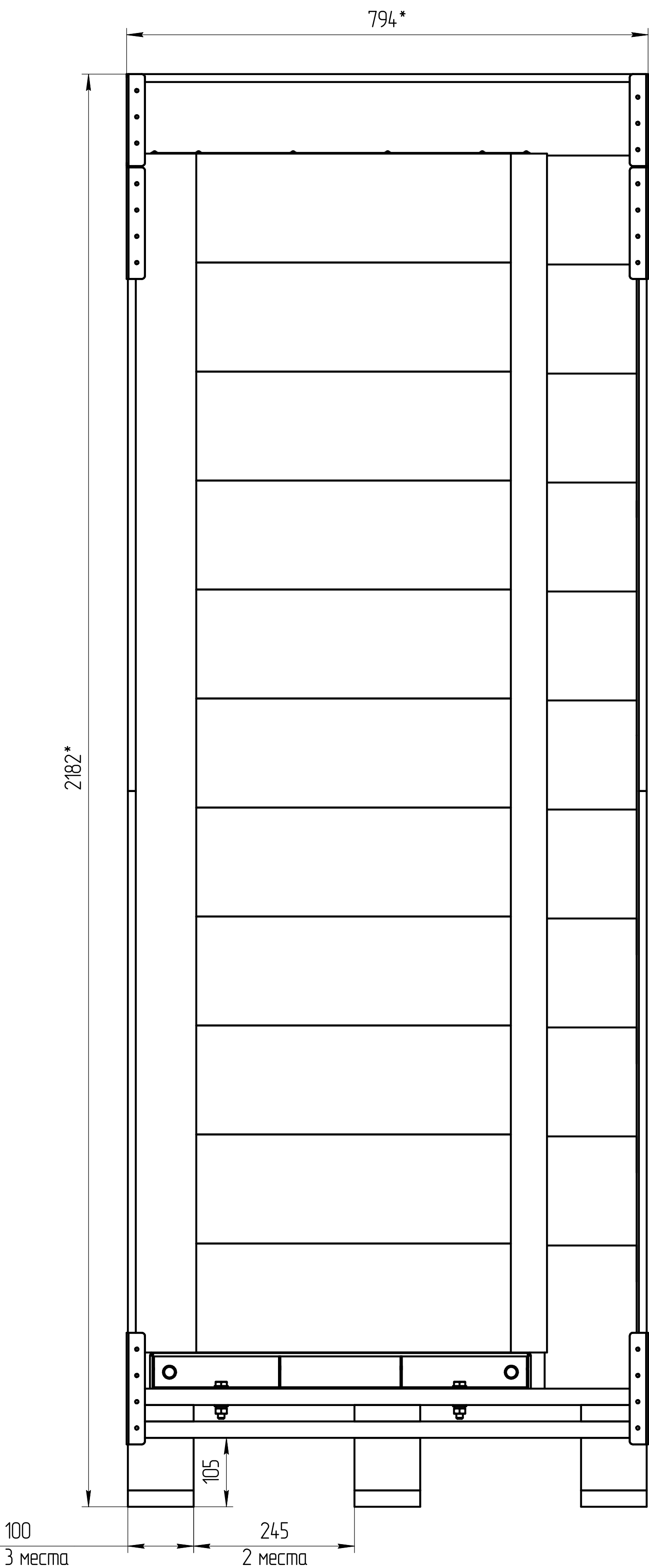
Вид сверху
