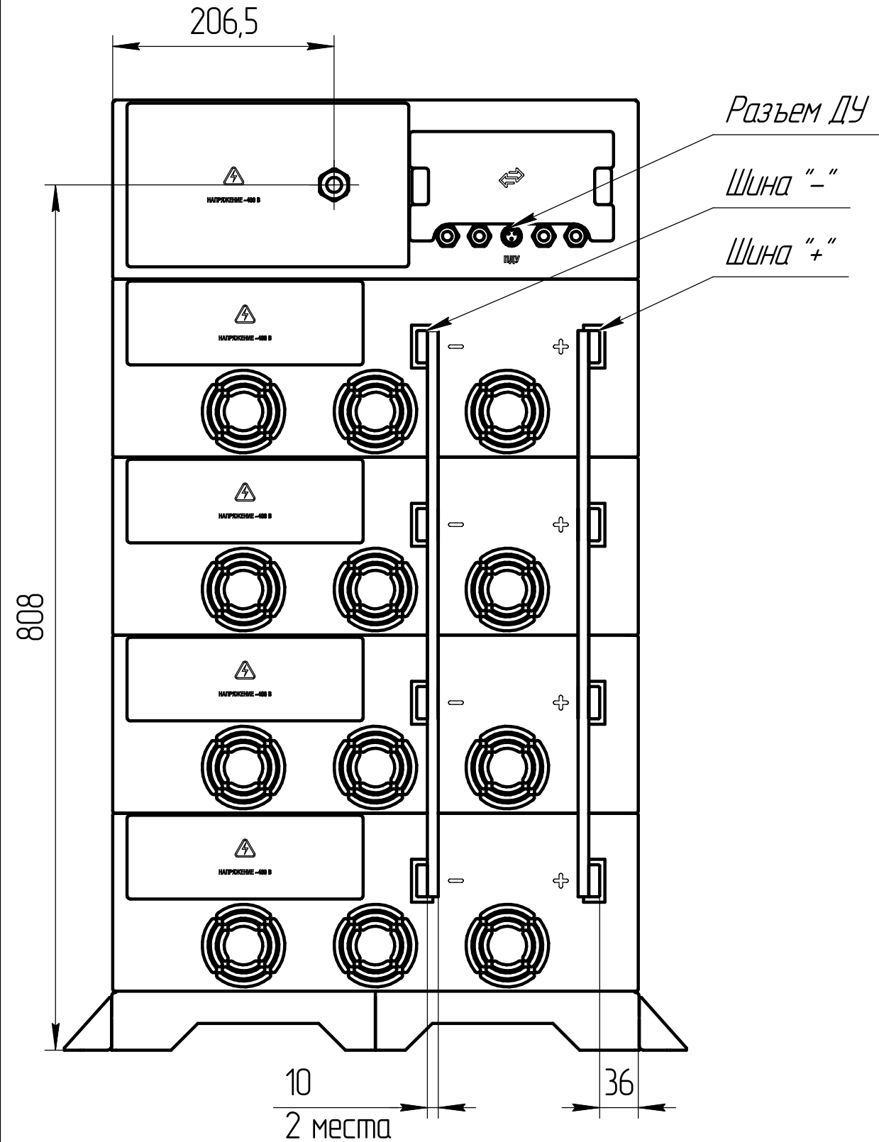
Вид сзади
