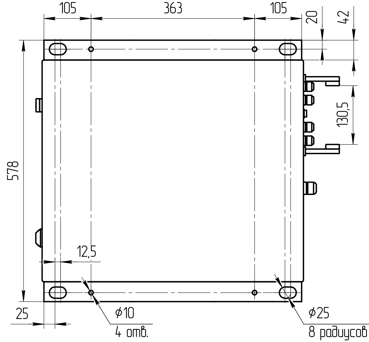
Вид сверху
