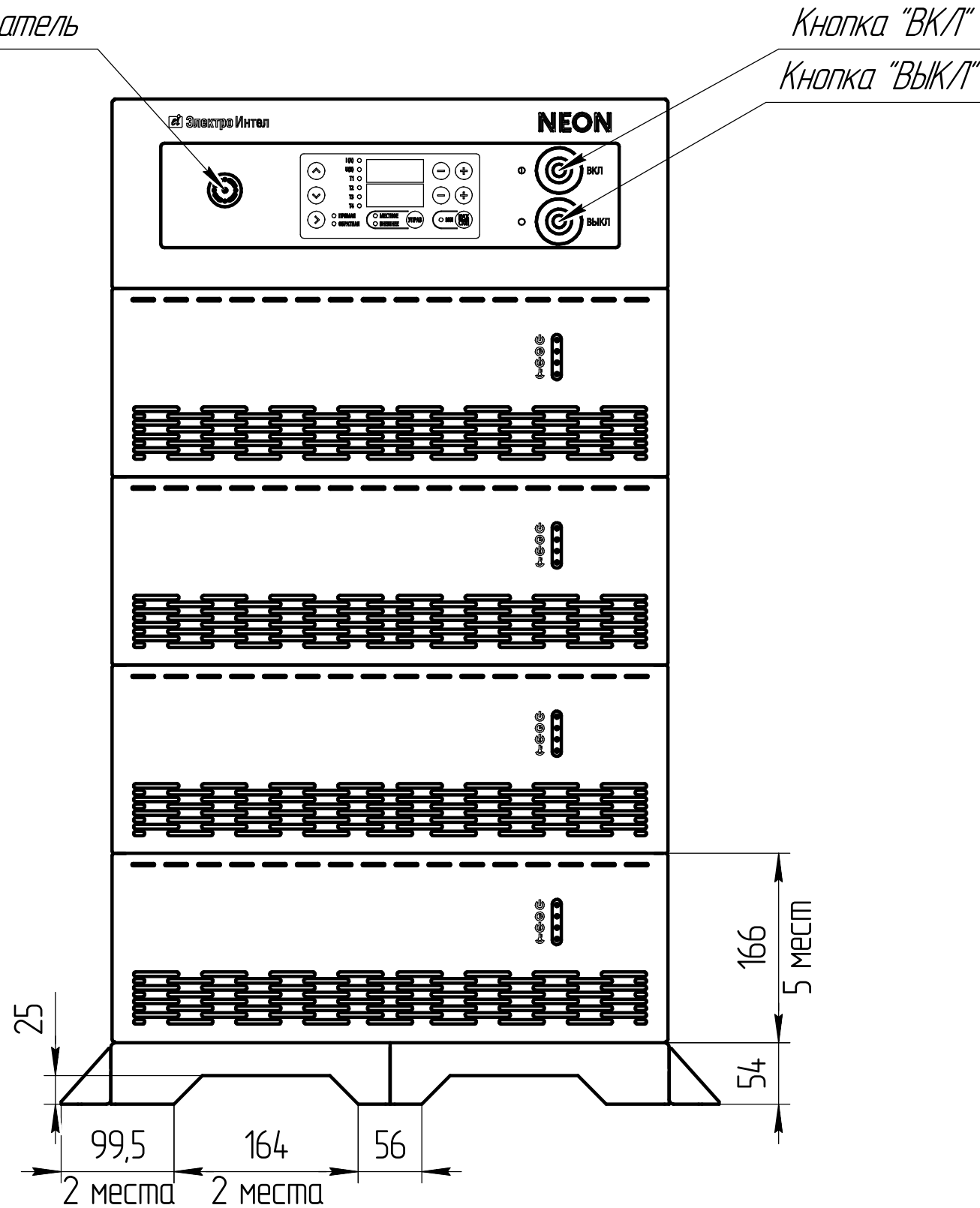
Вид спереди
