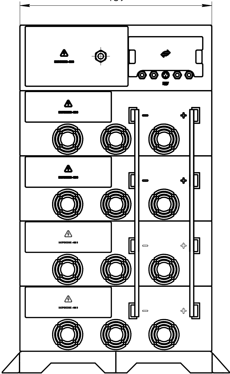
Вид сзади 489
