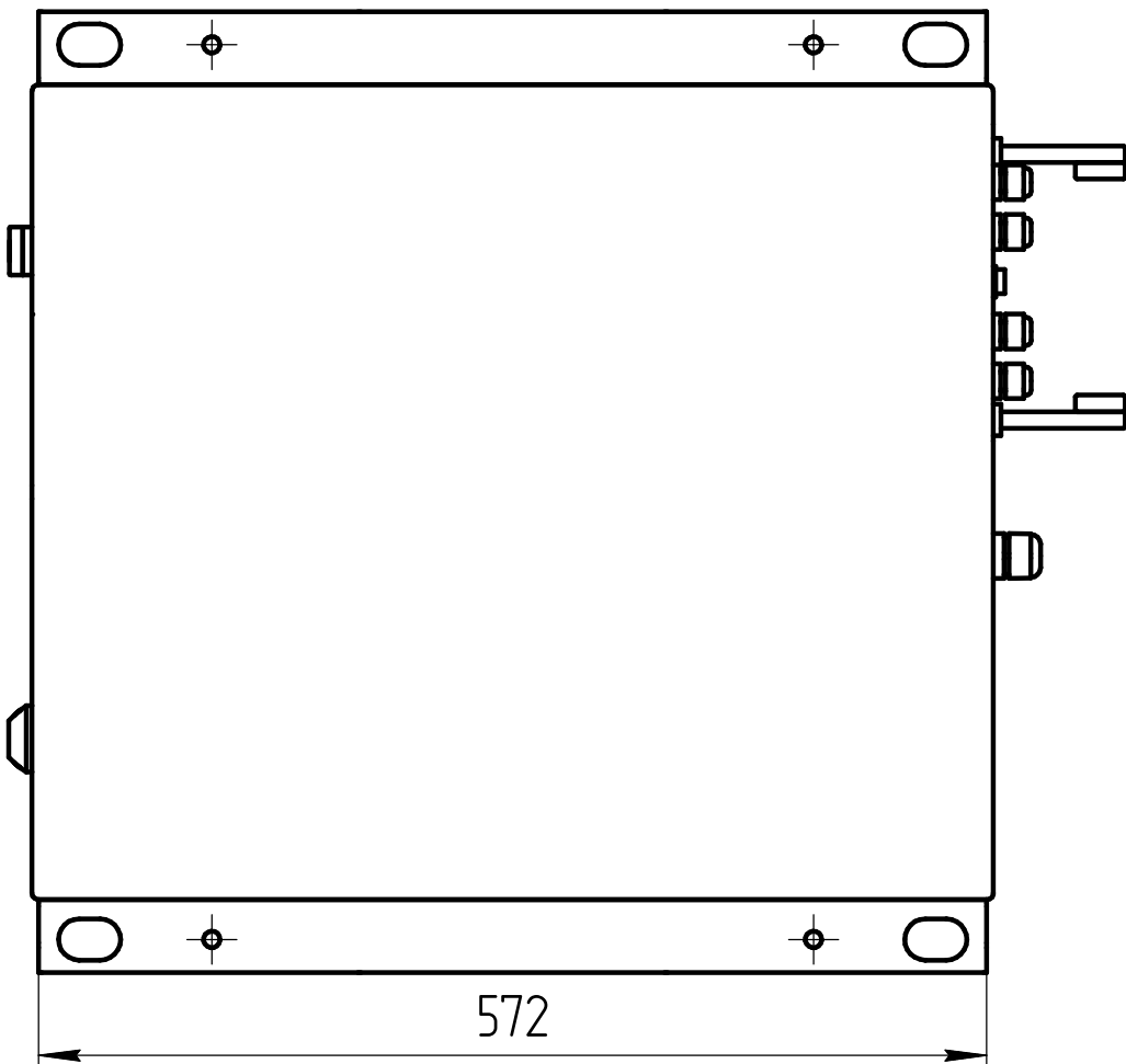
Вид сверху
