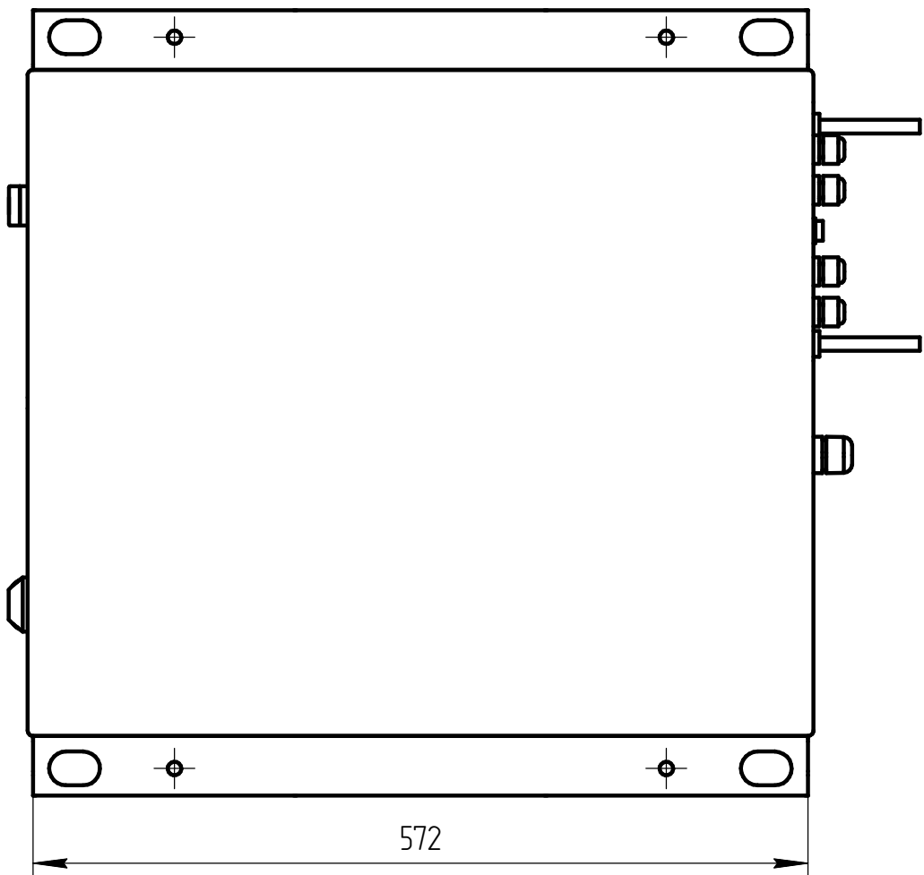
Вид сверху
