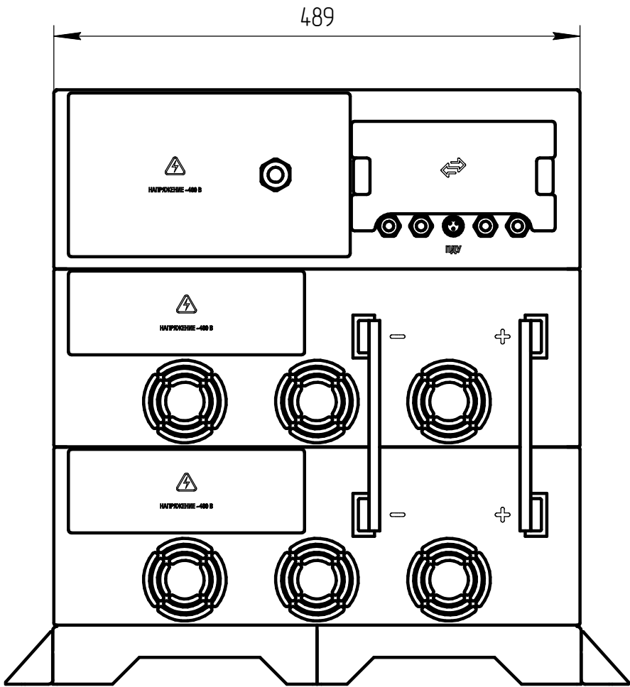
Вид сзади
