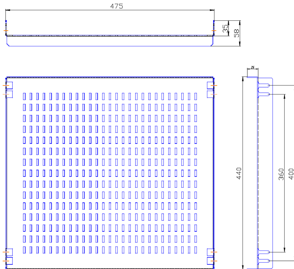
Рисунок 1 – Габаритные размеры полки стационарной Штиль FS-070-600
