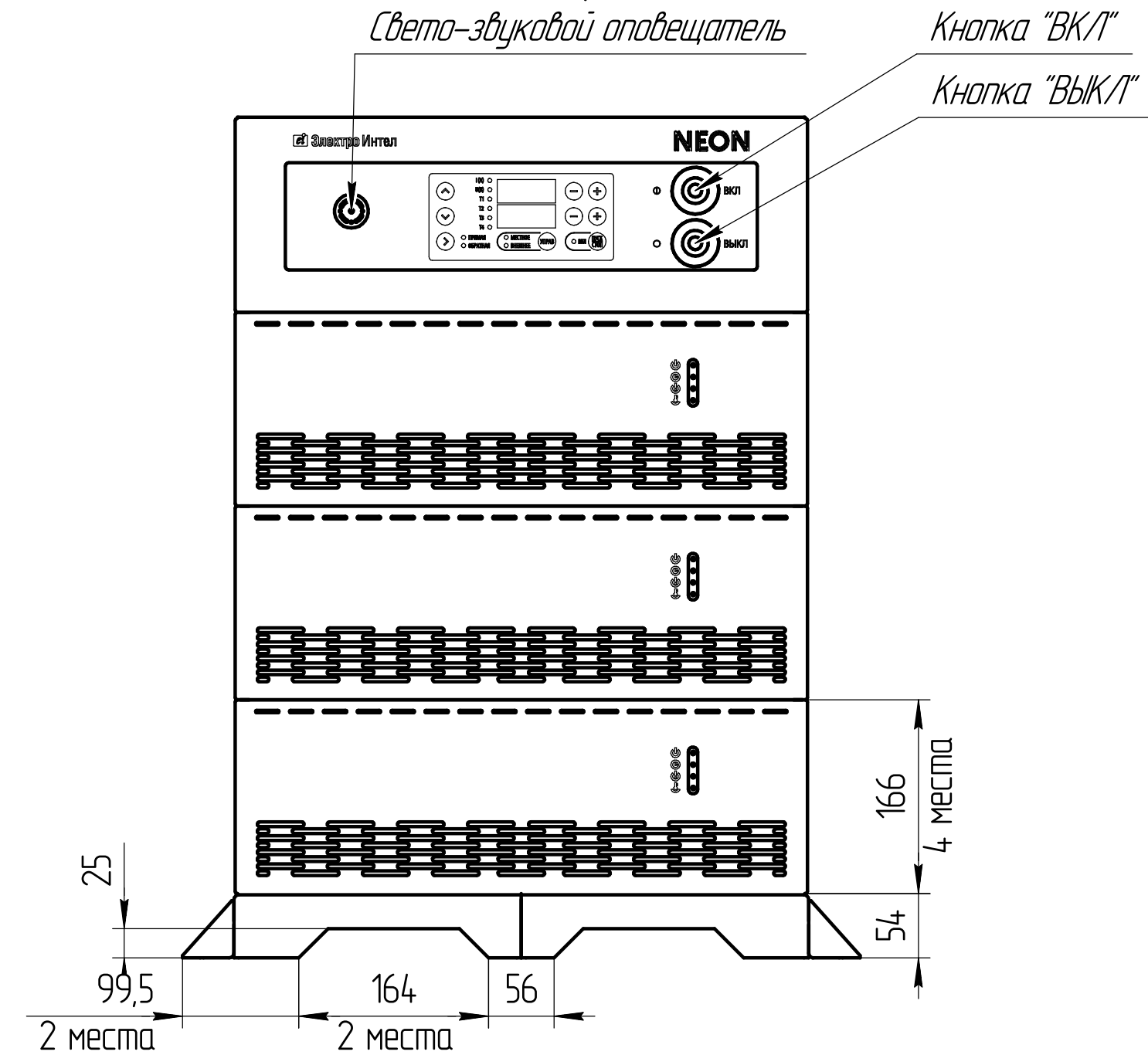
Вид спереди
