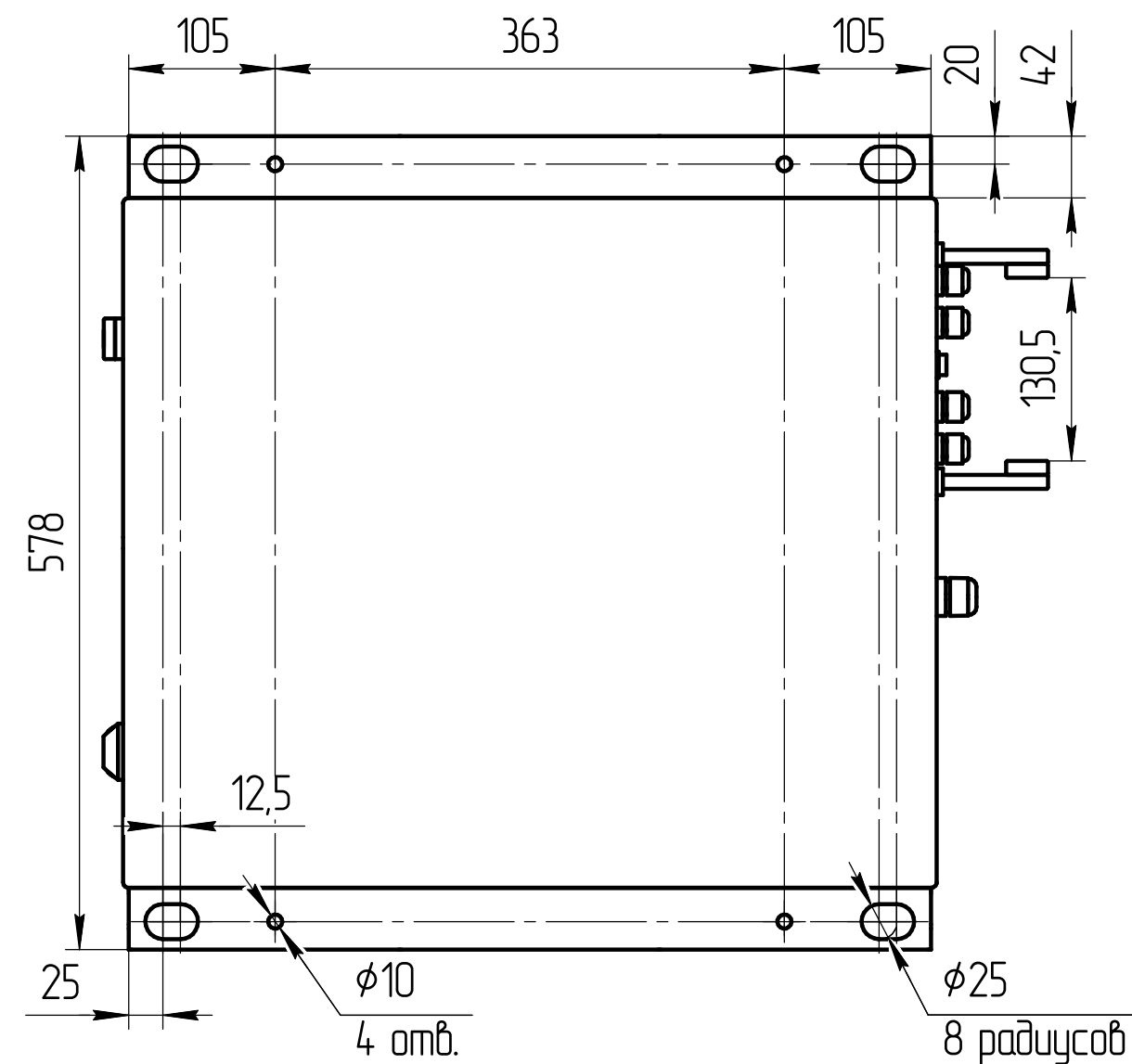
Вид сверху
