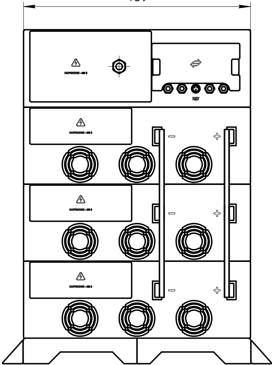
Вид сзади 489
