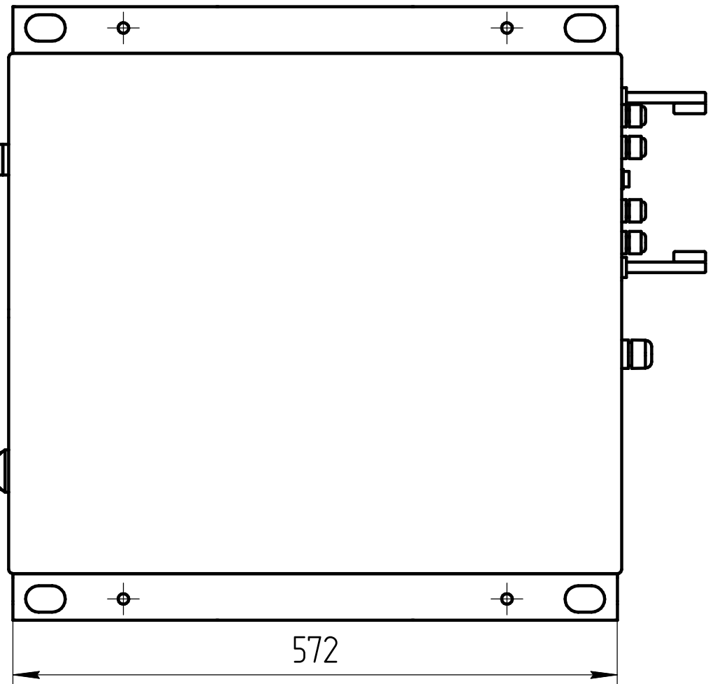
Вид сверху
