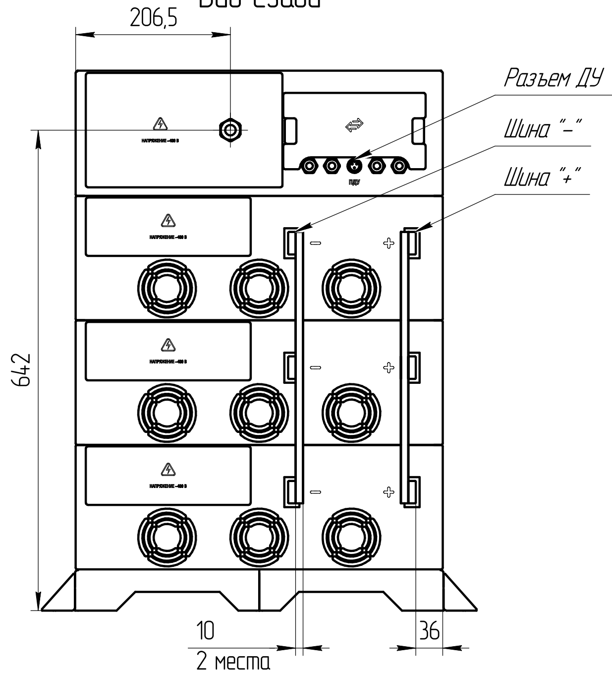
Вид сзади
