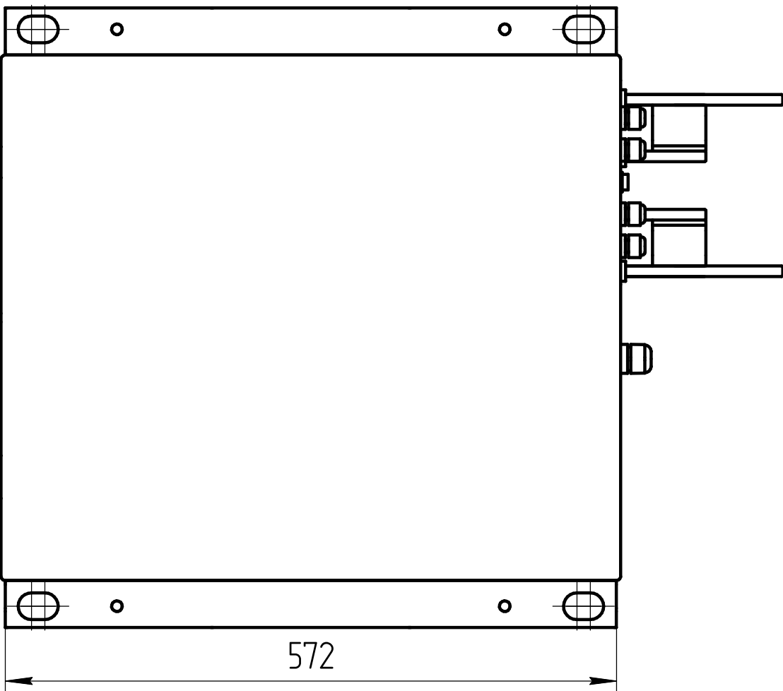
Вид сверху
