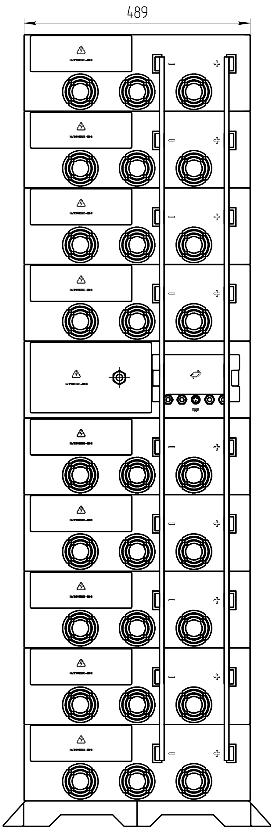
Вид сзади
