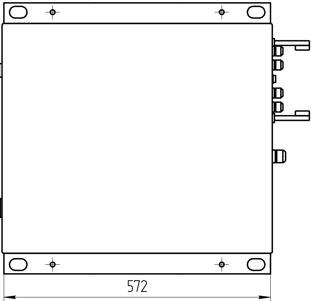
Вид сверху
