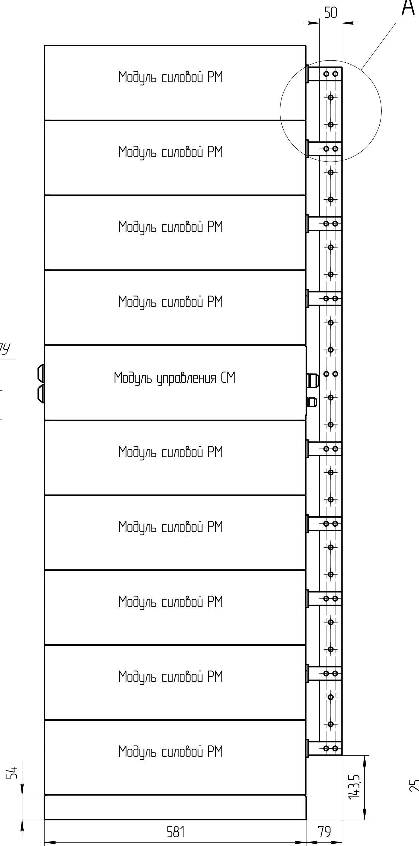
Вид сбоку
