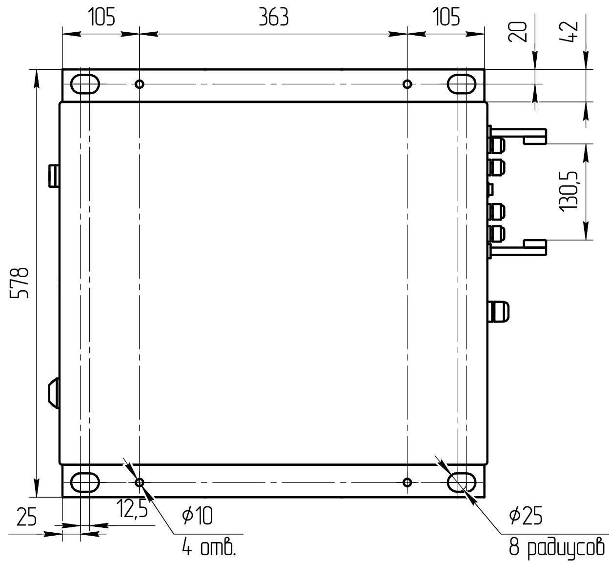
Вид сверху
