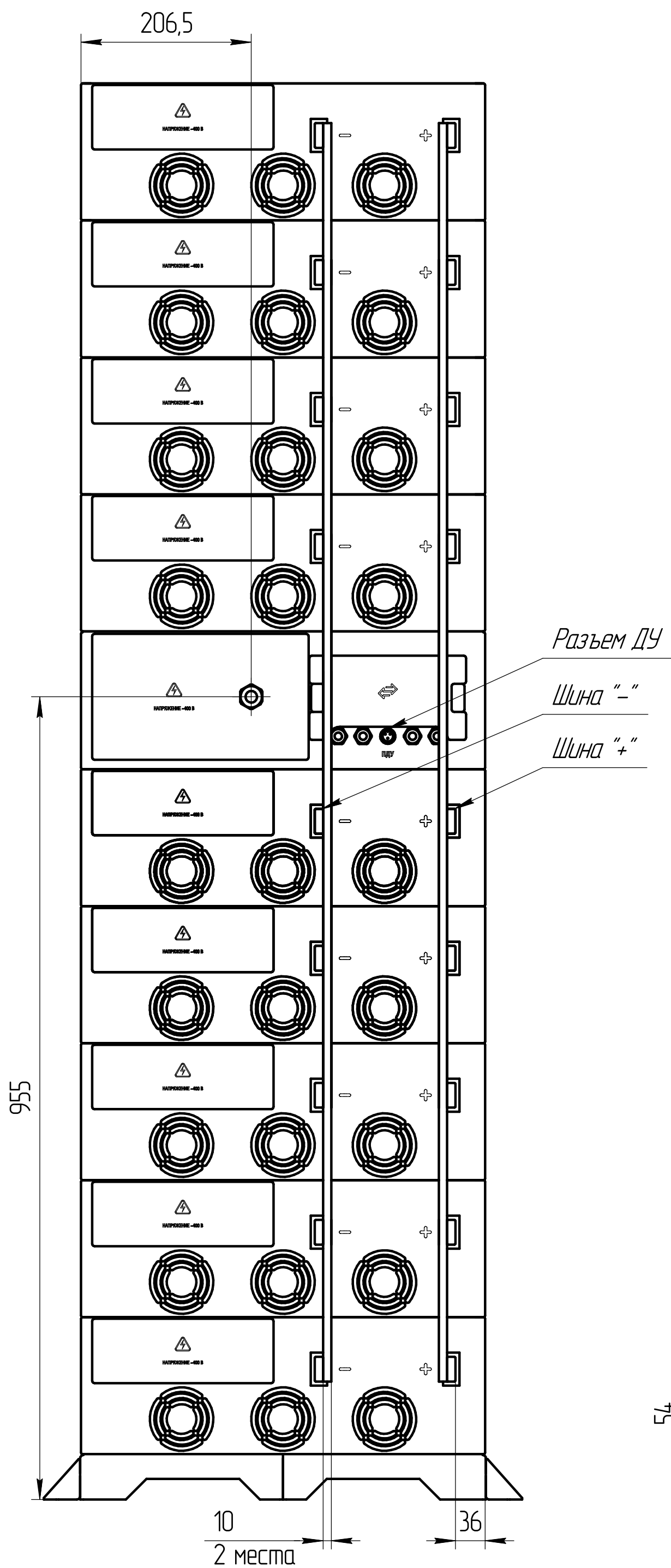
Вид сзади
