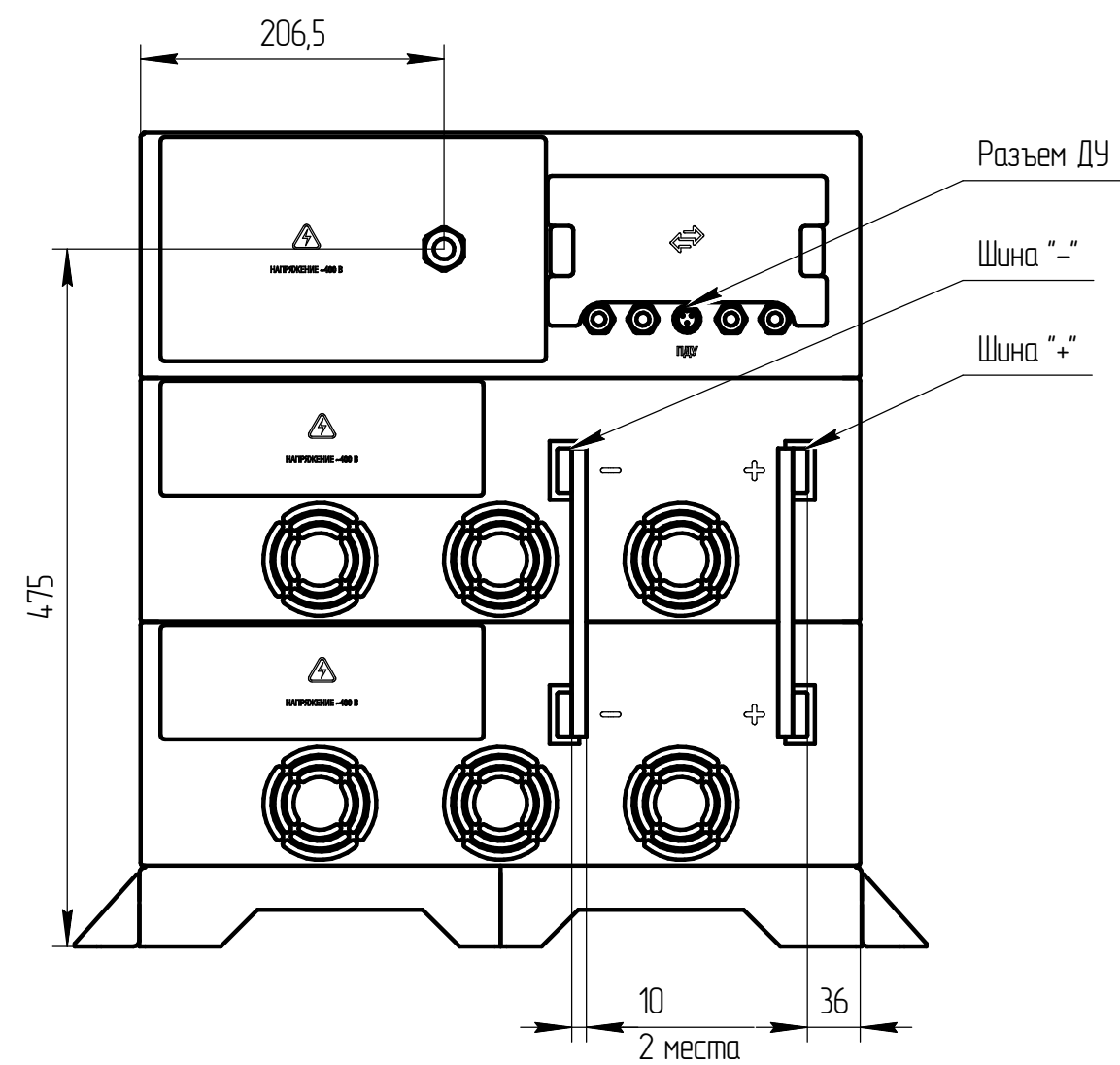
Вид сзади
