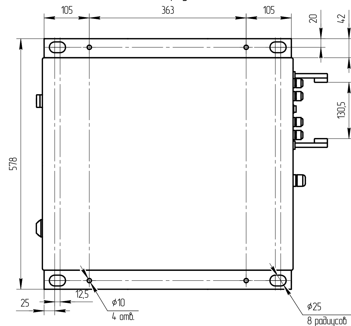
Вид сверху
