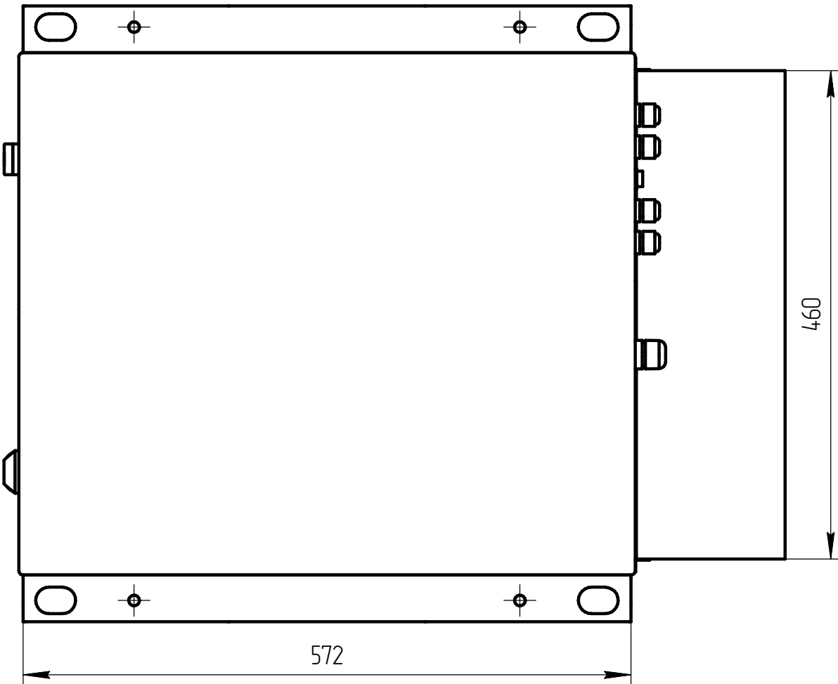
Вид сверху
