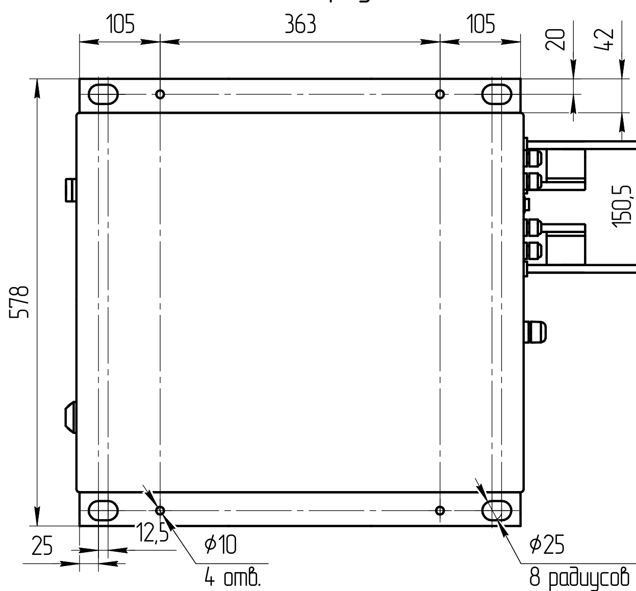
Вид сверху
