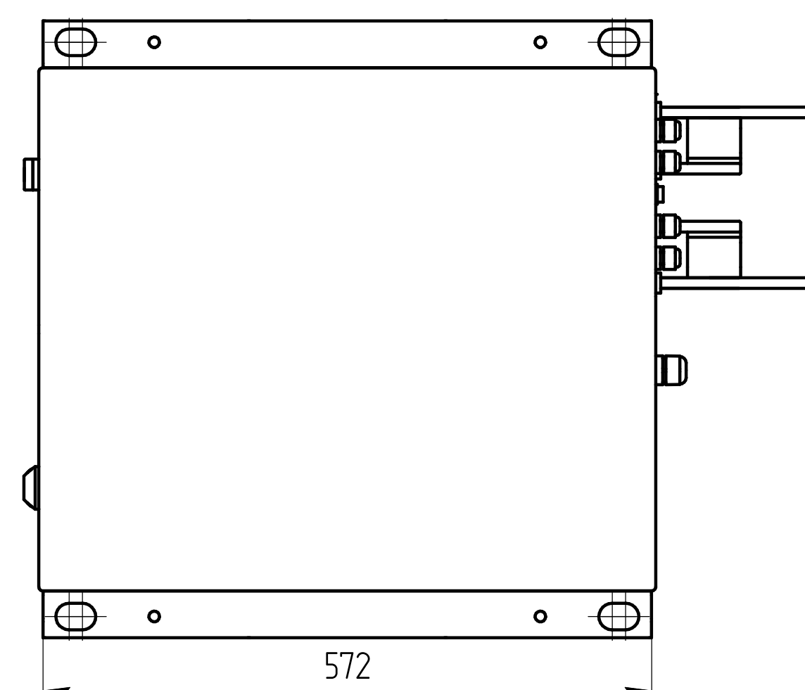
Вид сверху
