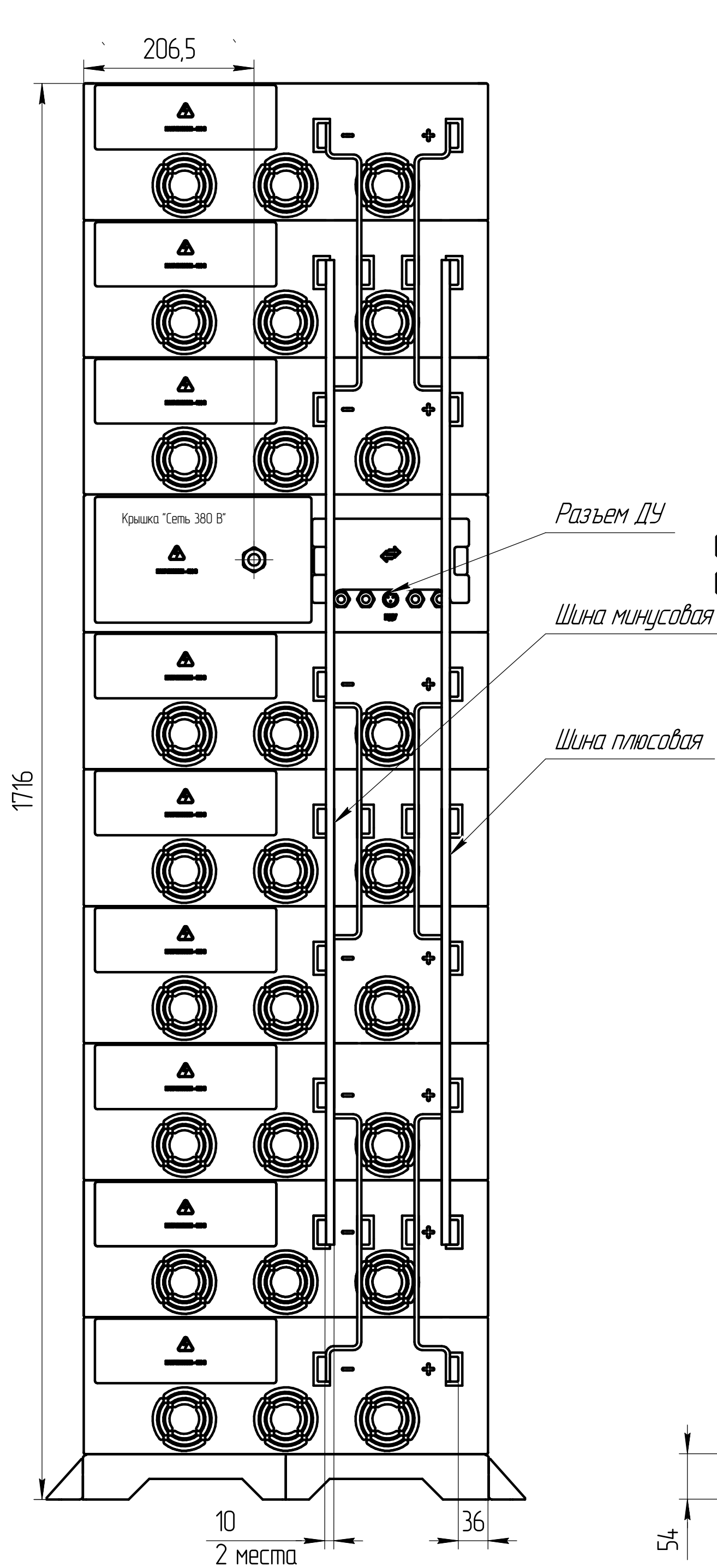
Вид сзади
