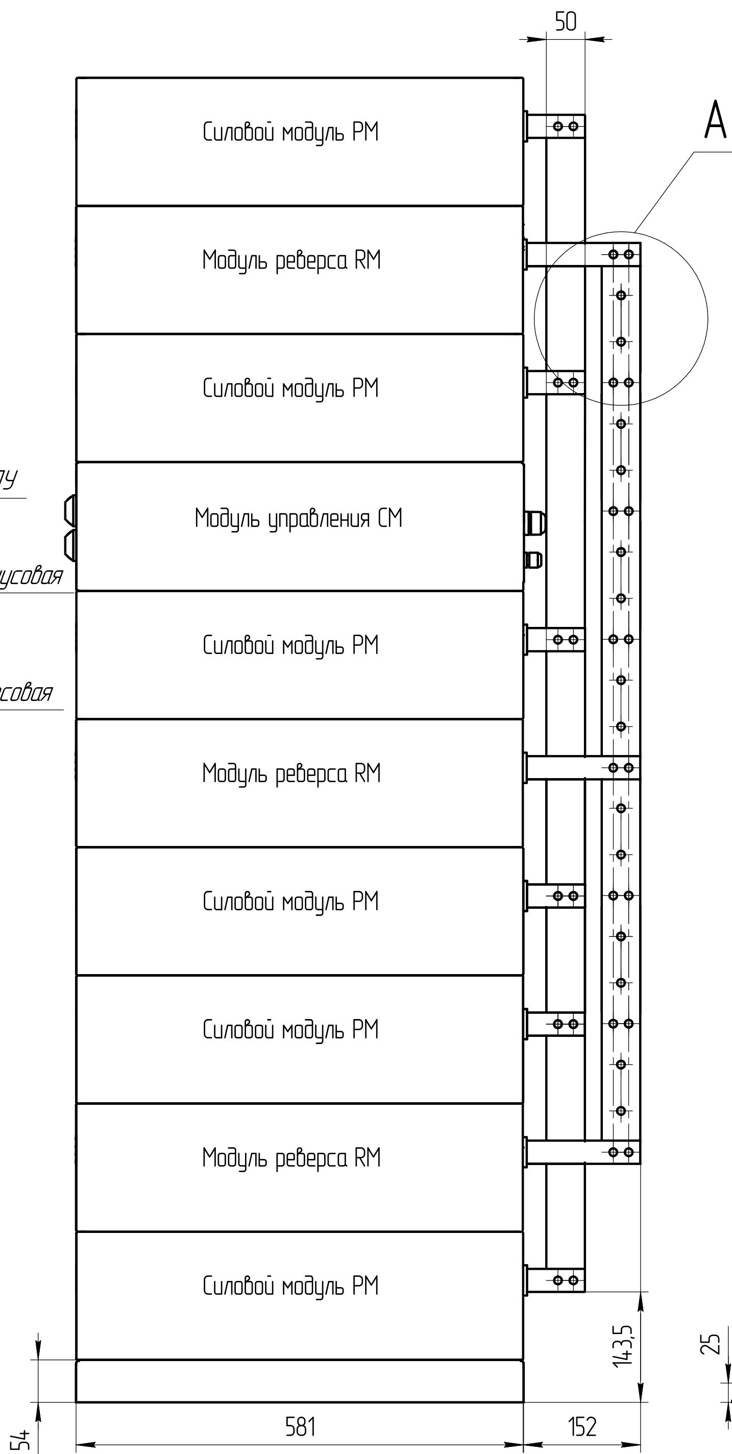
Вид сбоку
