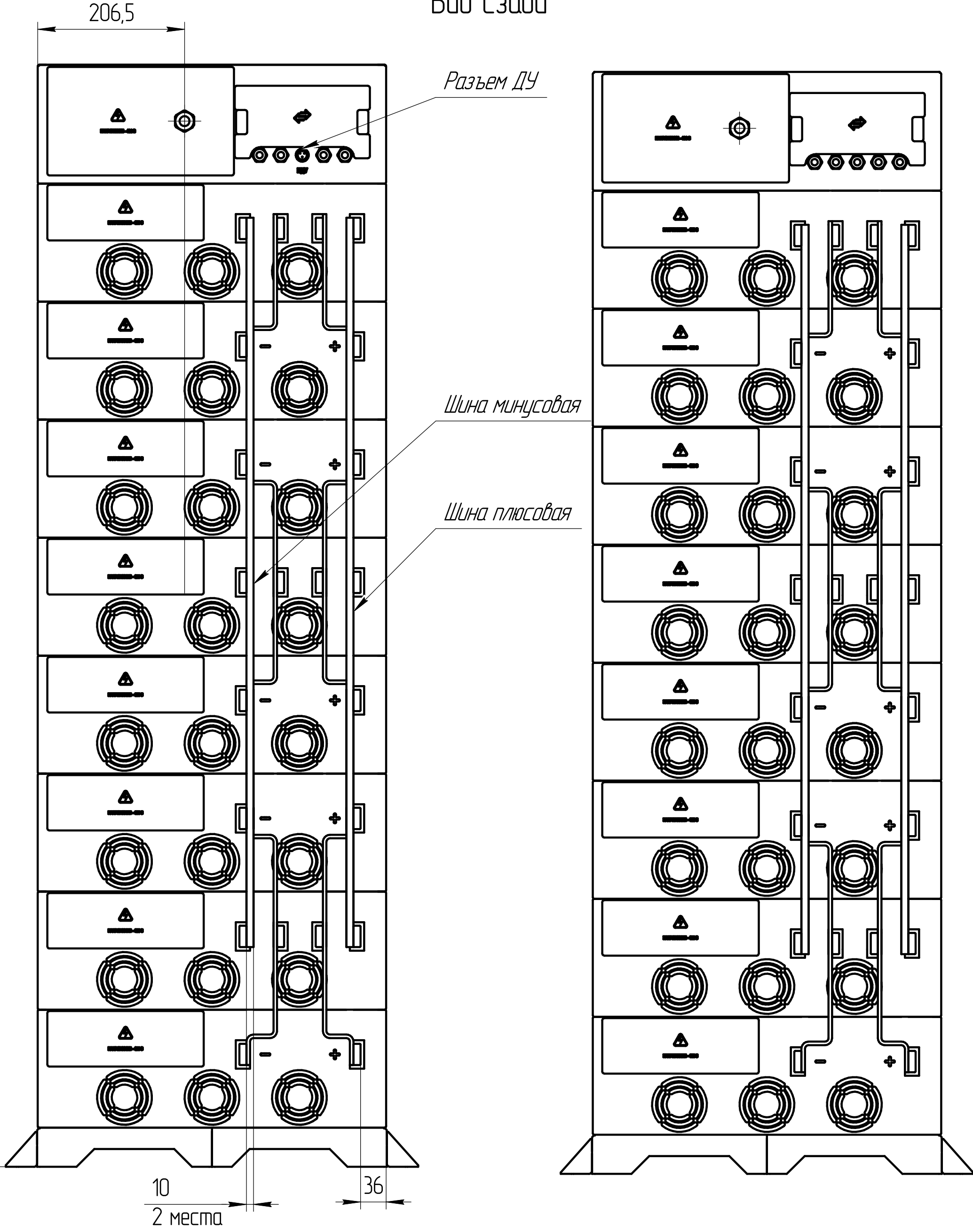
Вид сзади
