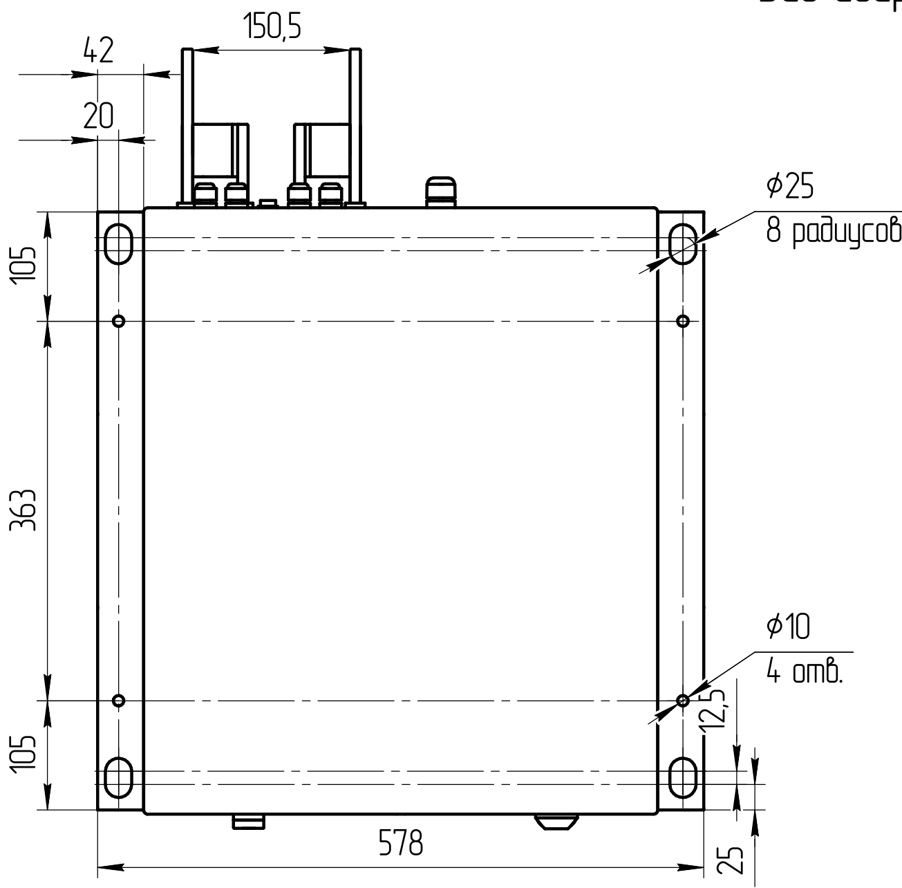
Вид сверху
