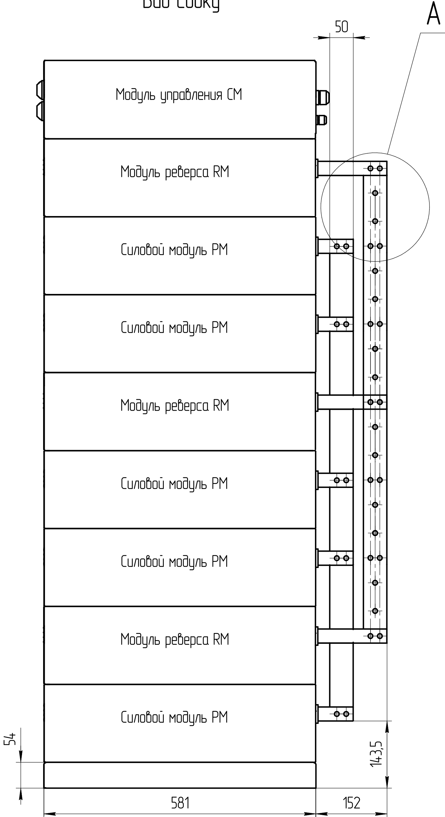
Вид сбоку
