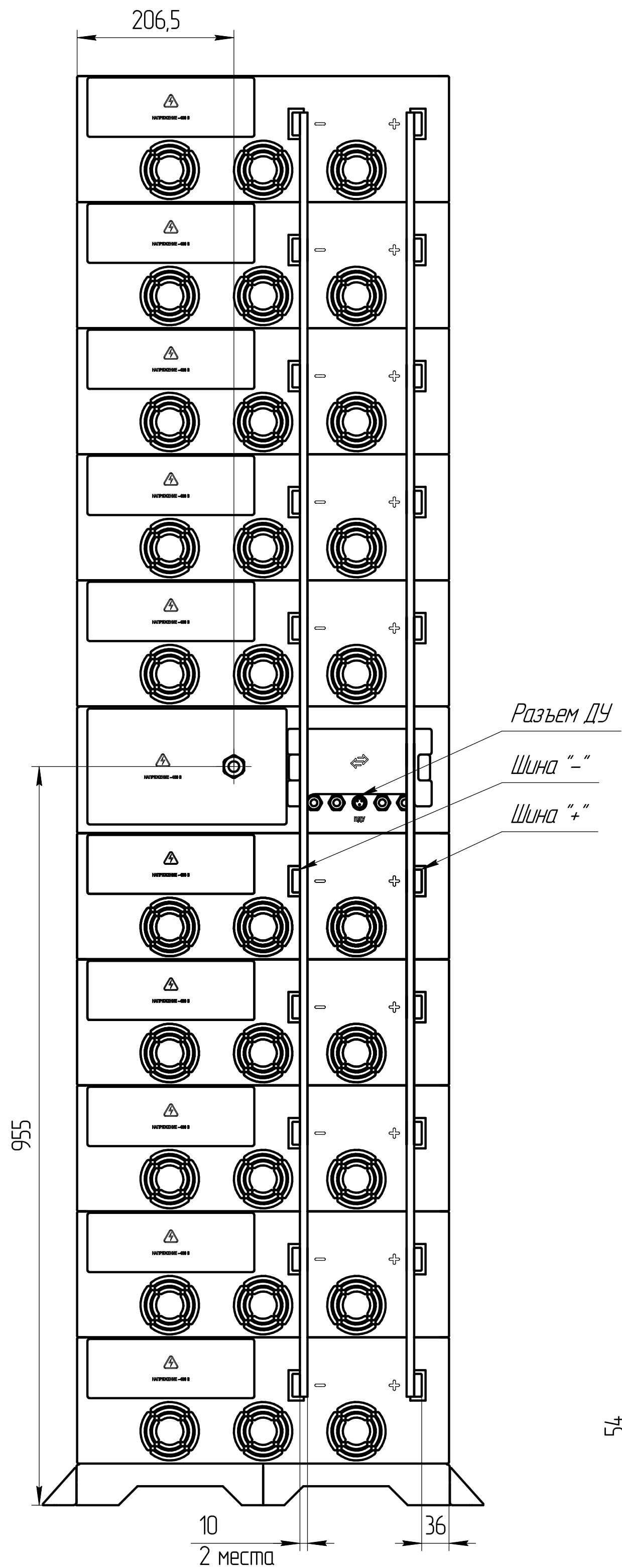
Вид сзади
