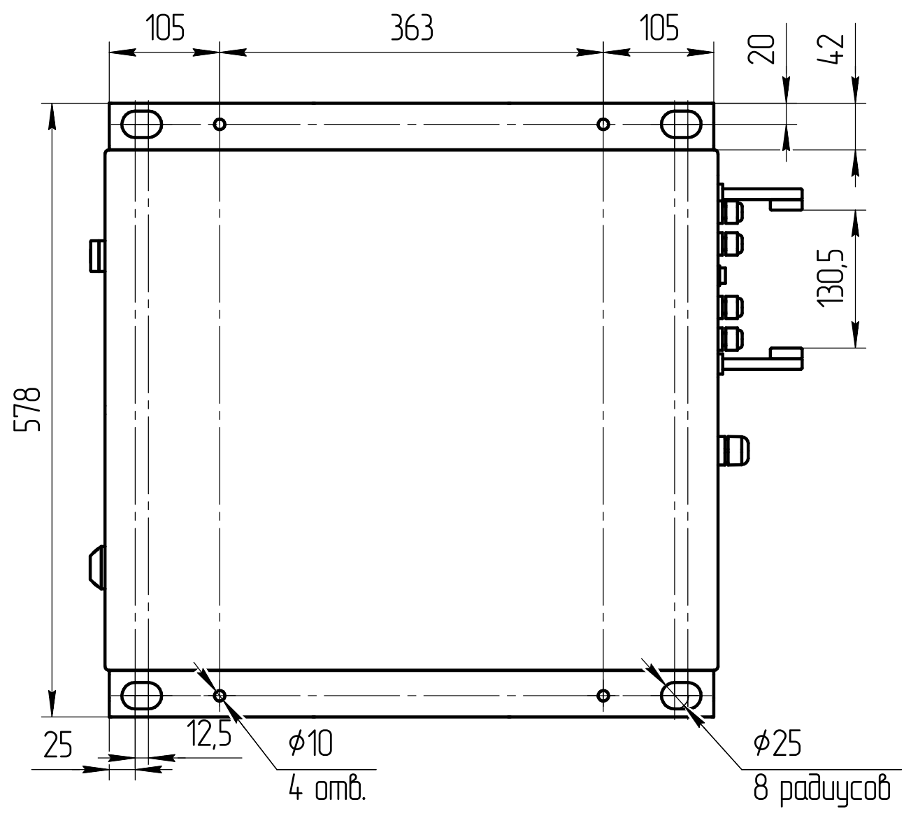
Вид сверху
