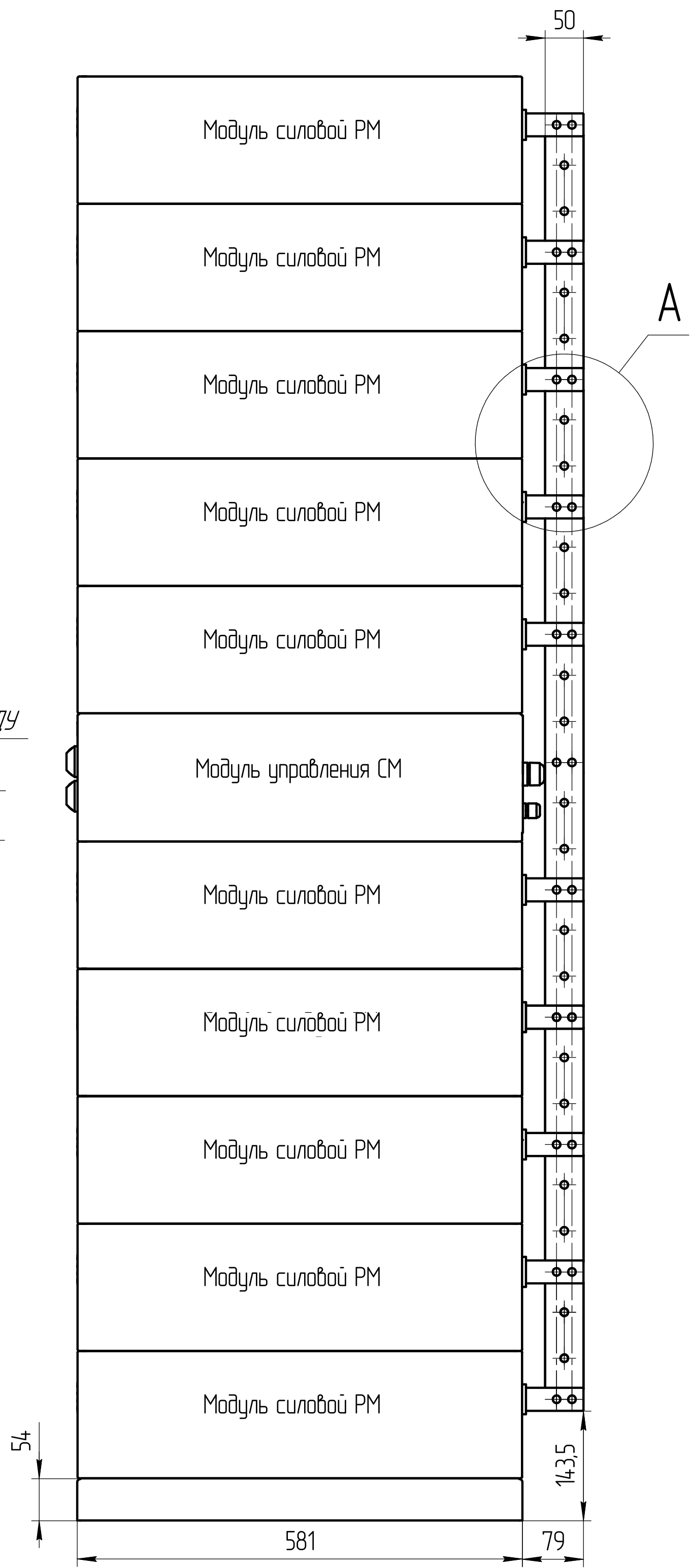
Вид сверху
