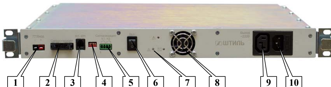
Рисунок 1.1 - Инвертор Штиль PS48-60/500
