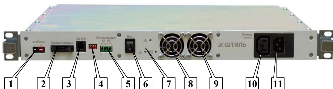
Рисунок 1.3- Инвертор Штиль PS48-60/1000
