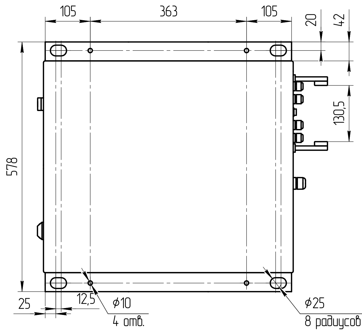
Вид сверху
