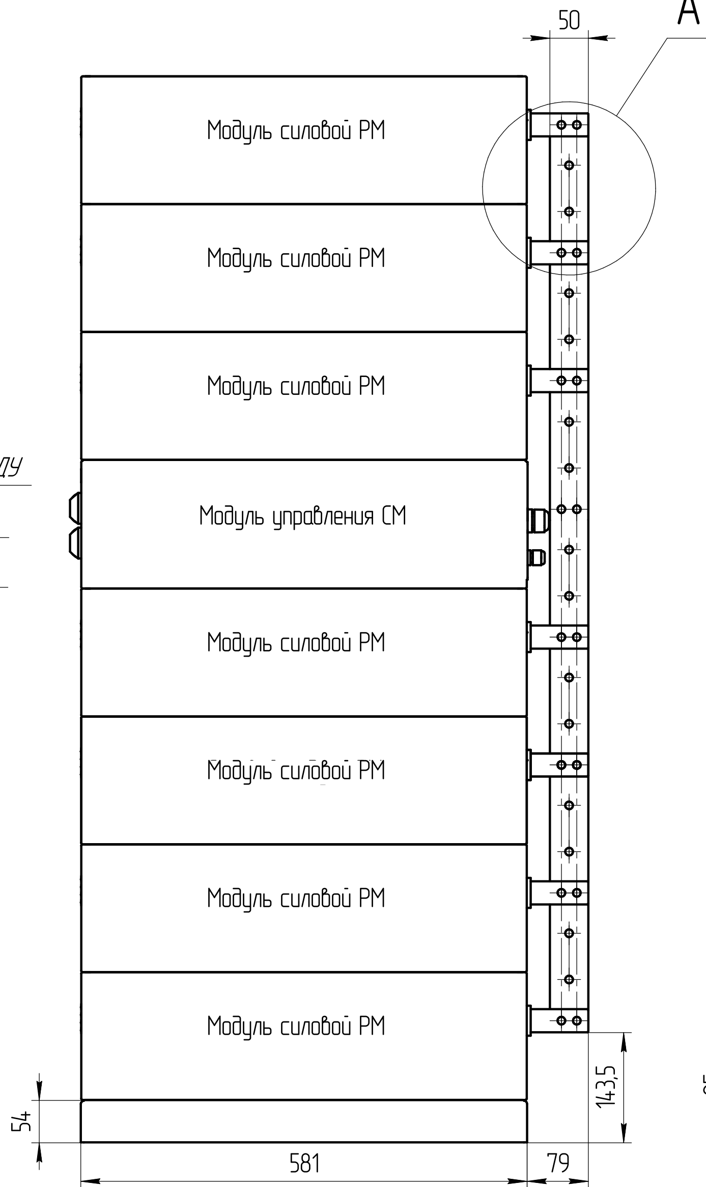
Вид сбоку
