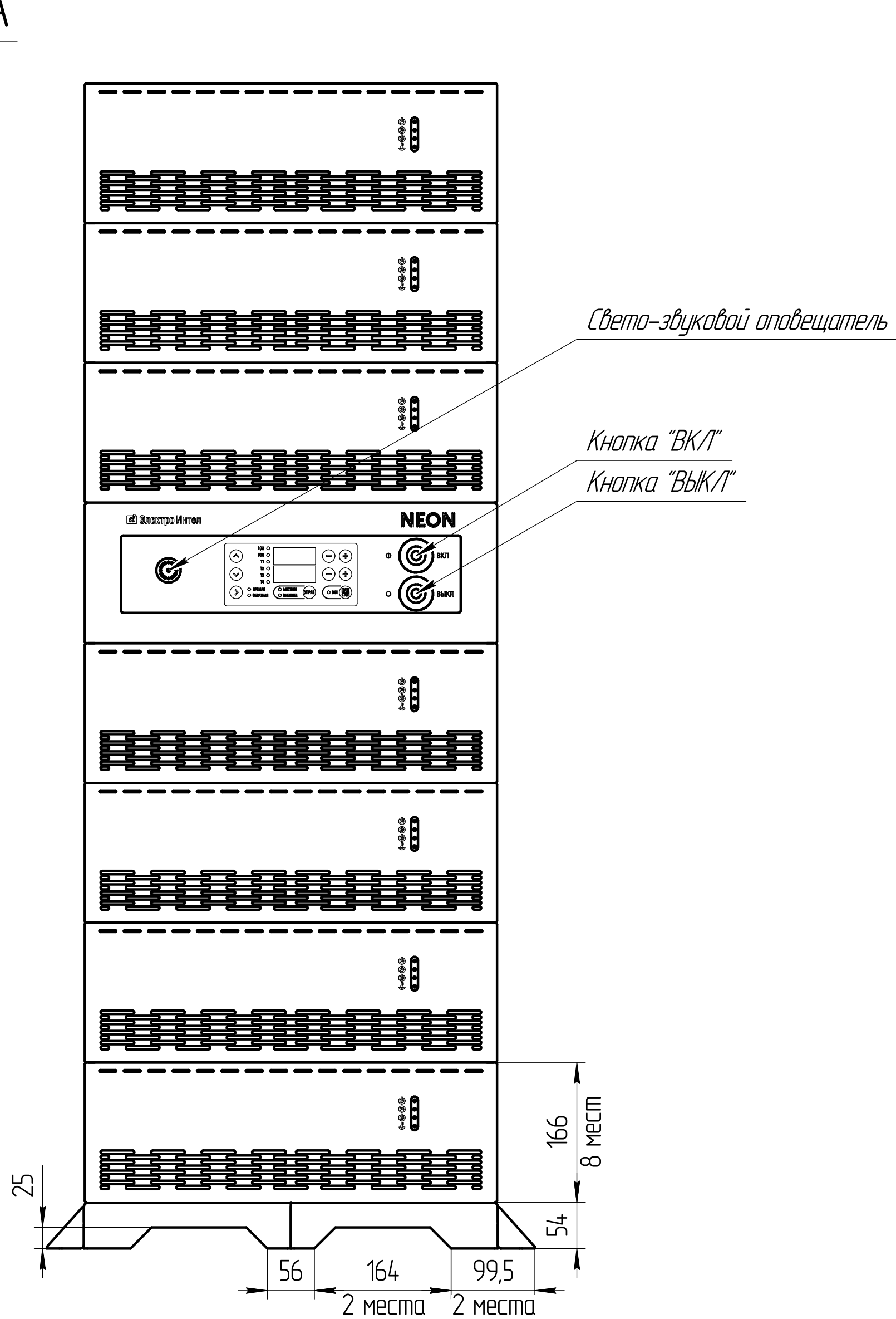
Вид спереди
