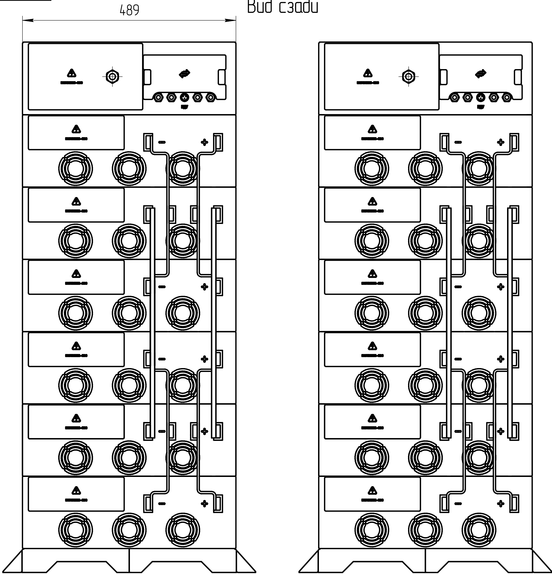
Вид сзади
