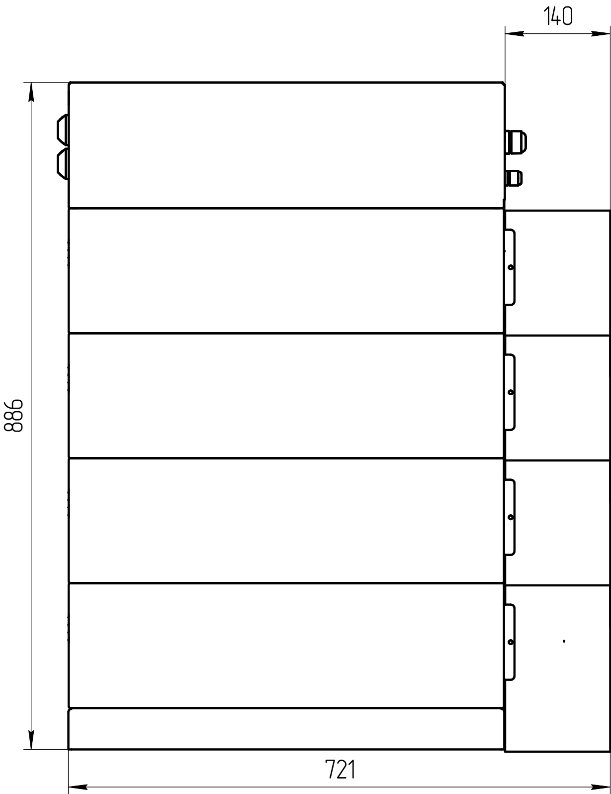
Вид сбоку
