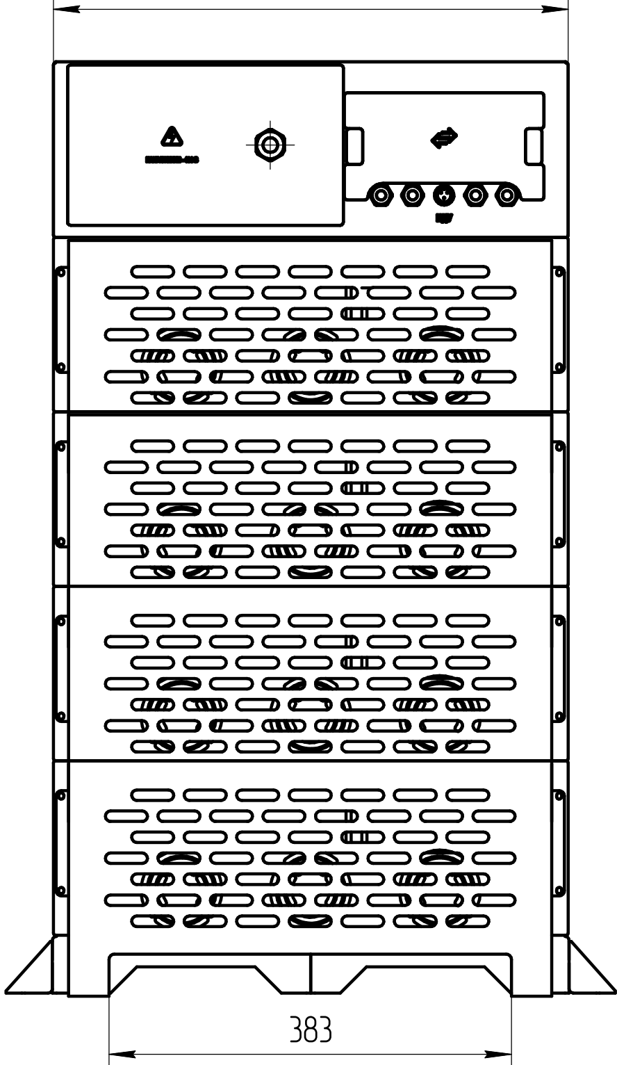
Вид сзади
