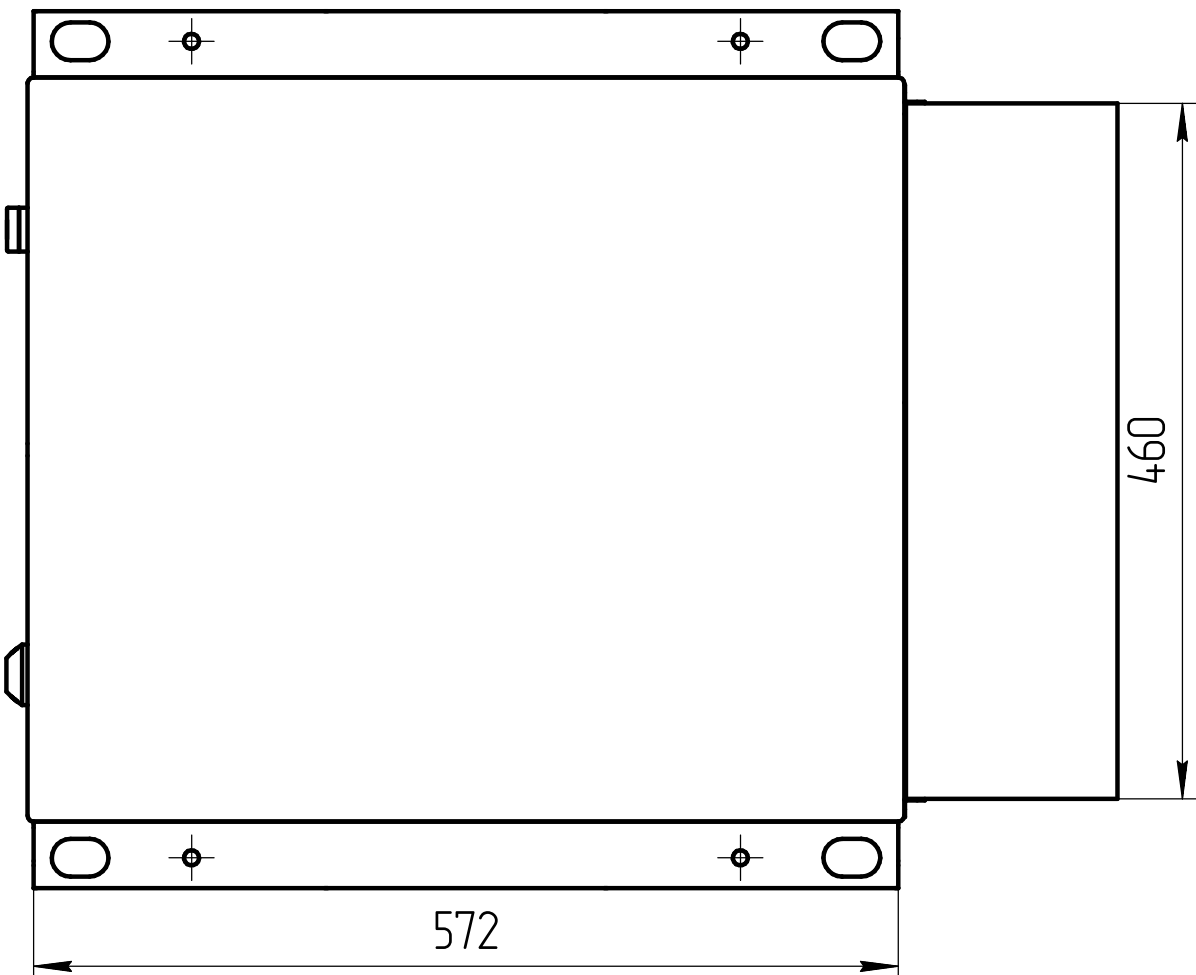
Вид сверху
