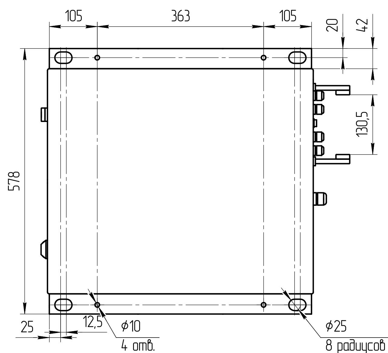
Вид сверху
