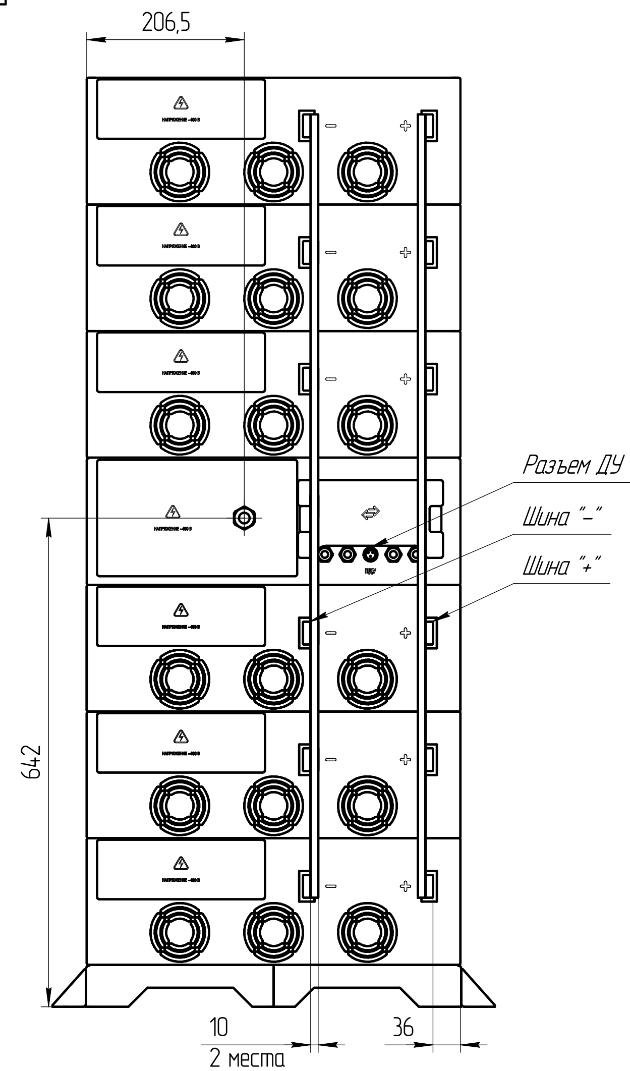
Види сзадѹ
