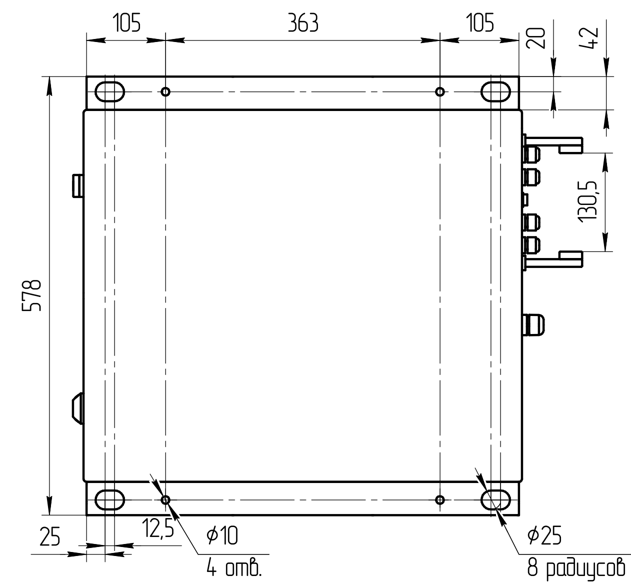
Вид сверху
