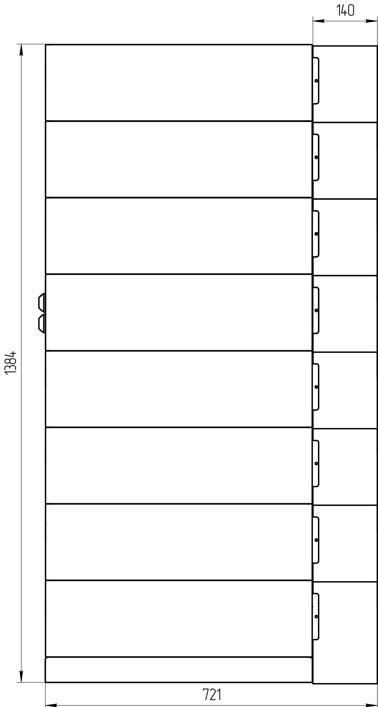
Вид сбоку
