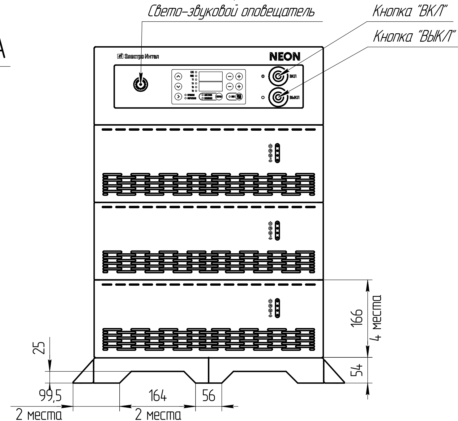
Вид спереди
