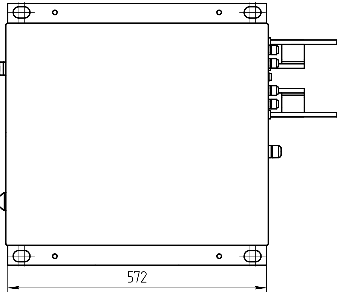
Вид сверху
