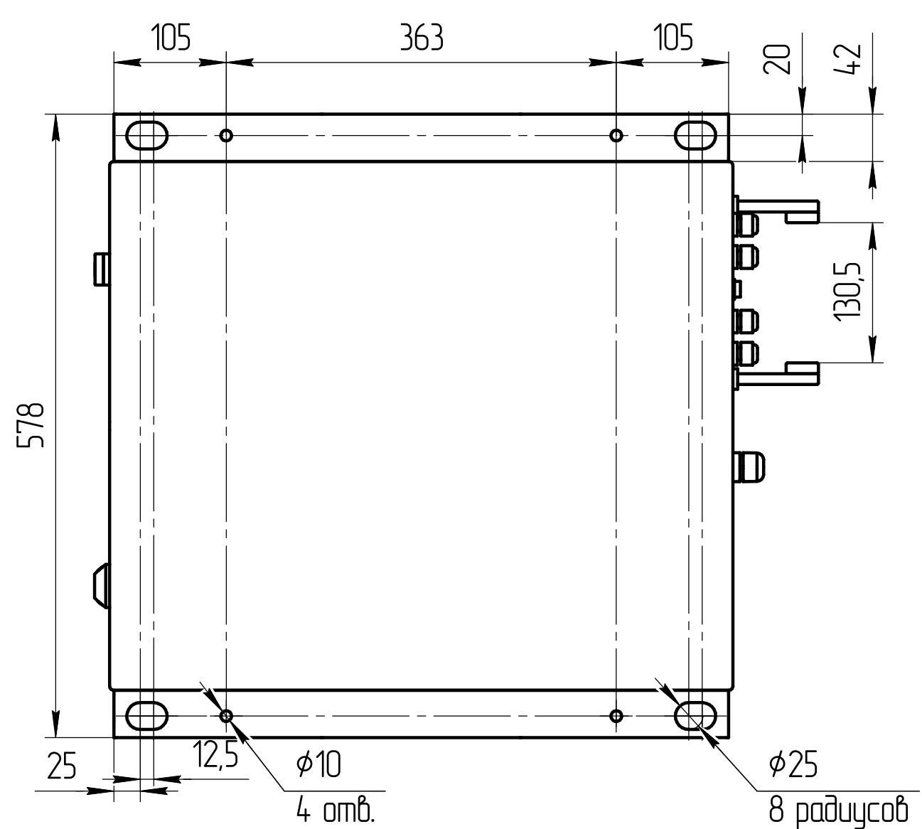
Вид сверху
