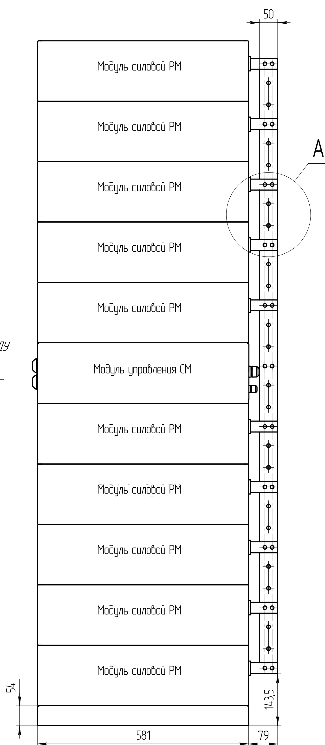
Вид сверху
