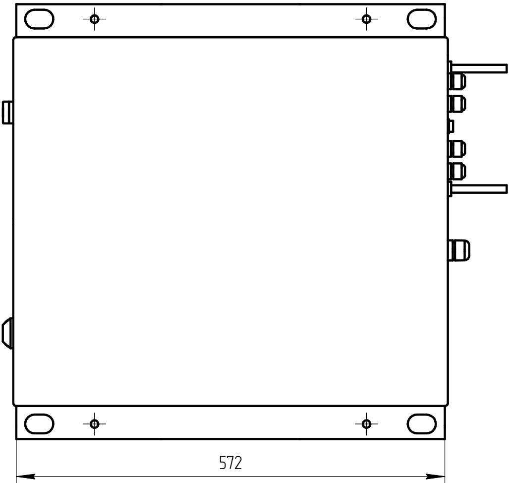
Вид сверху
