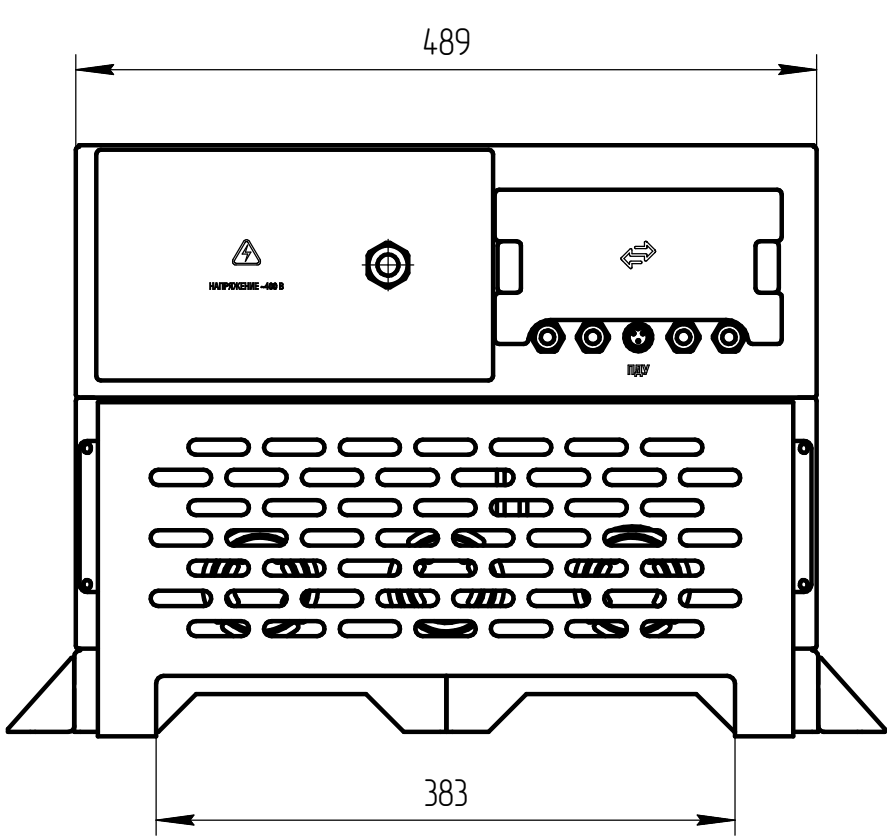
Вид сзади
