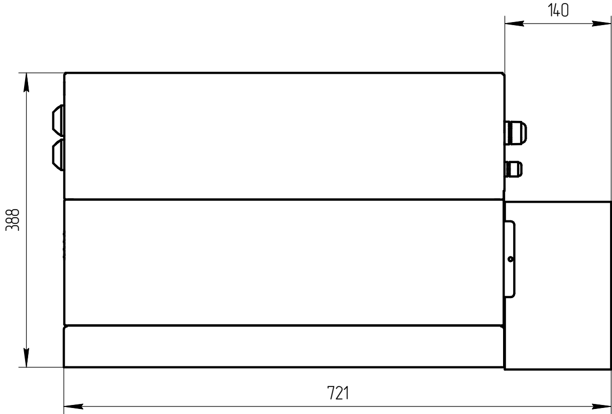
Вид сбоку
