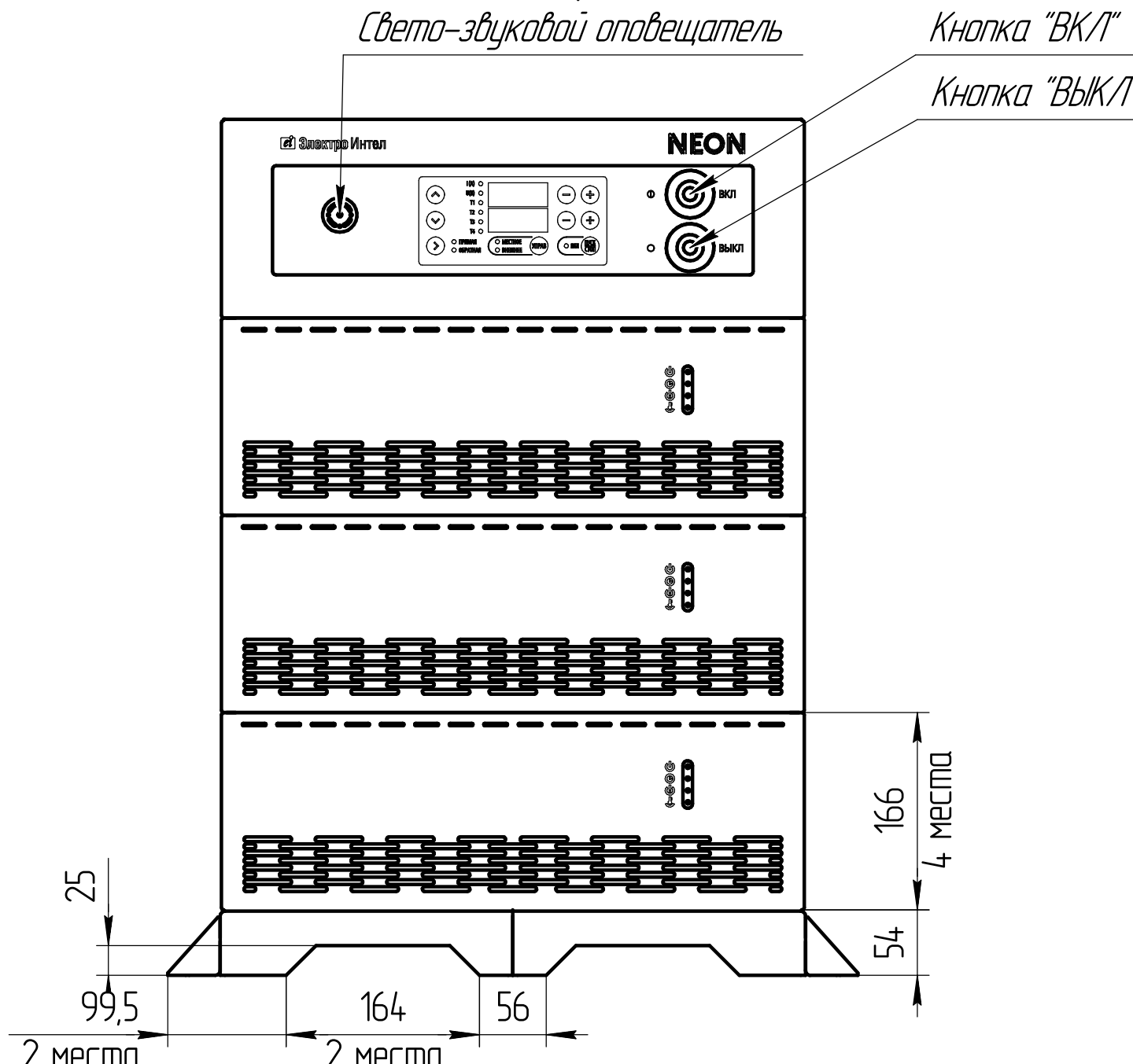
Вид спереди
