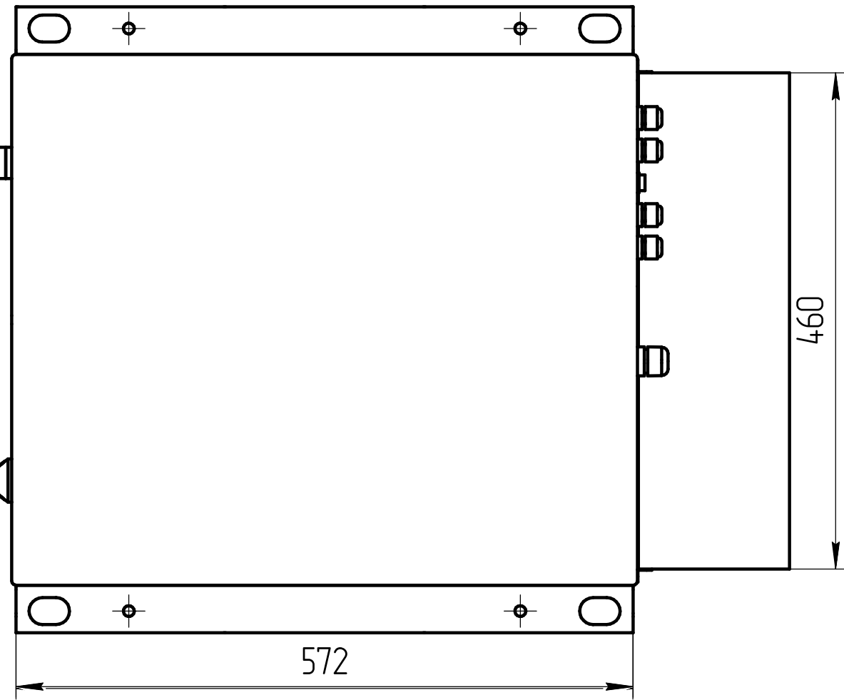
Вид сверху
