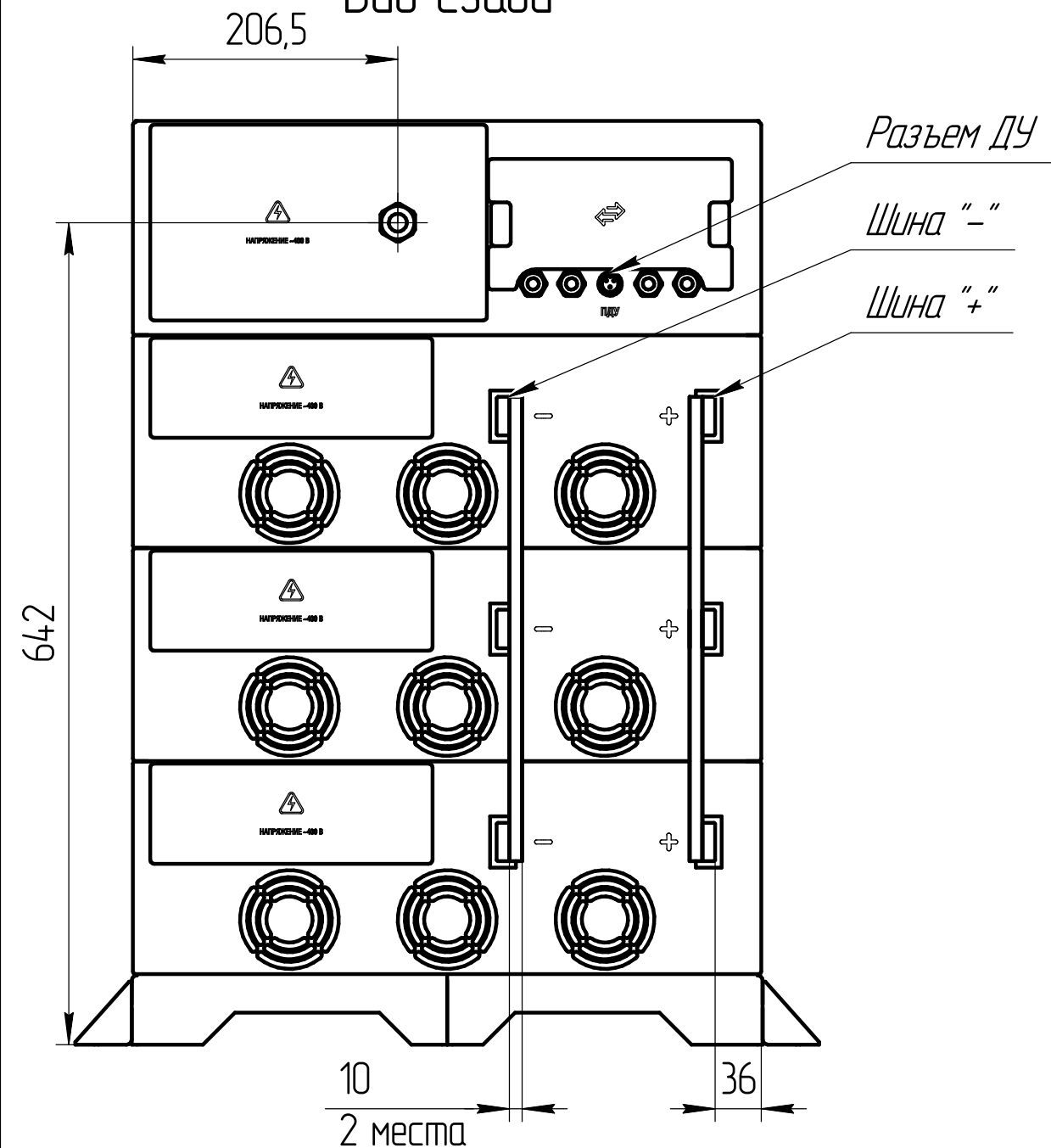
Вид сзади
