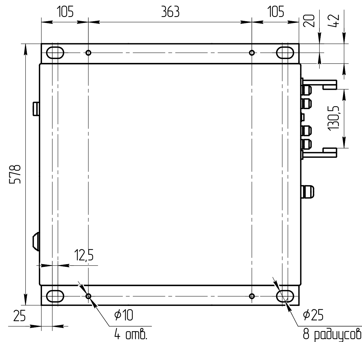
Вид сверху
