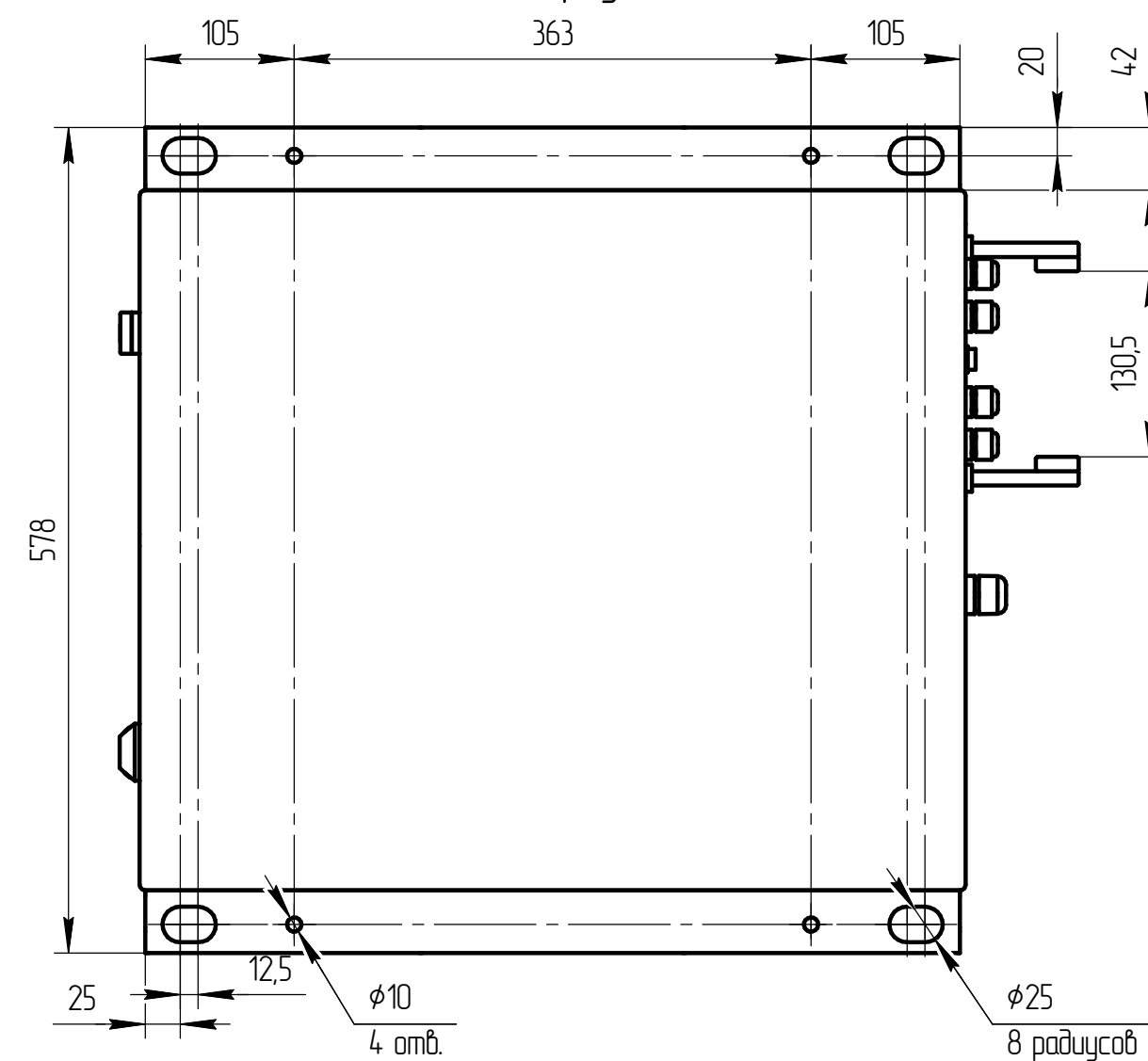
Вид сверху
