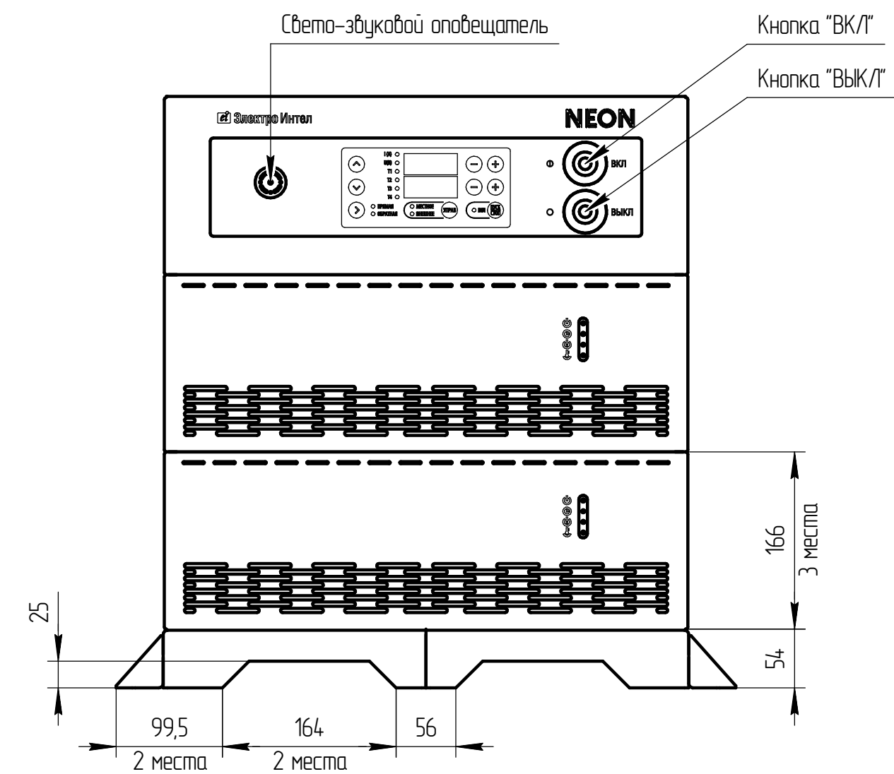
Вуд спереду
