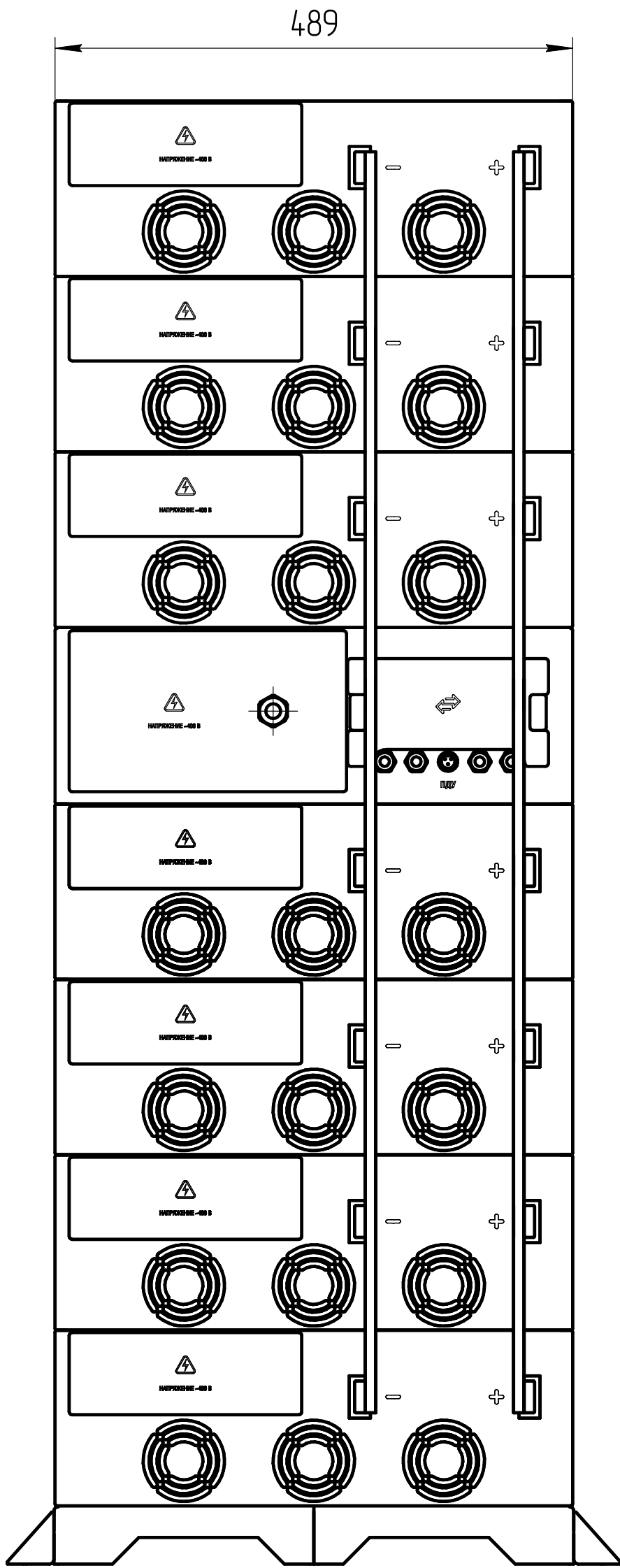
Вид сзади
