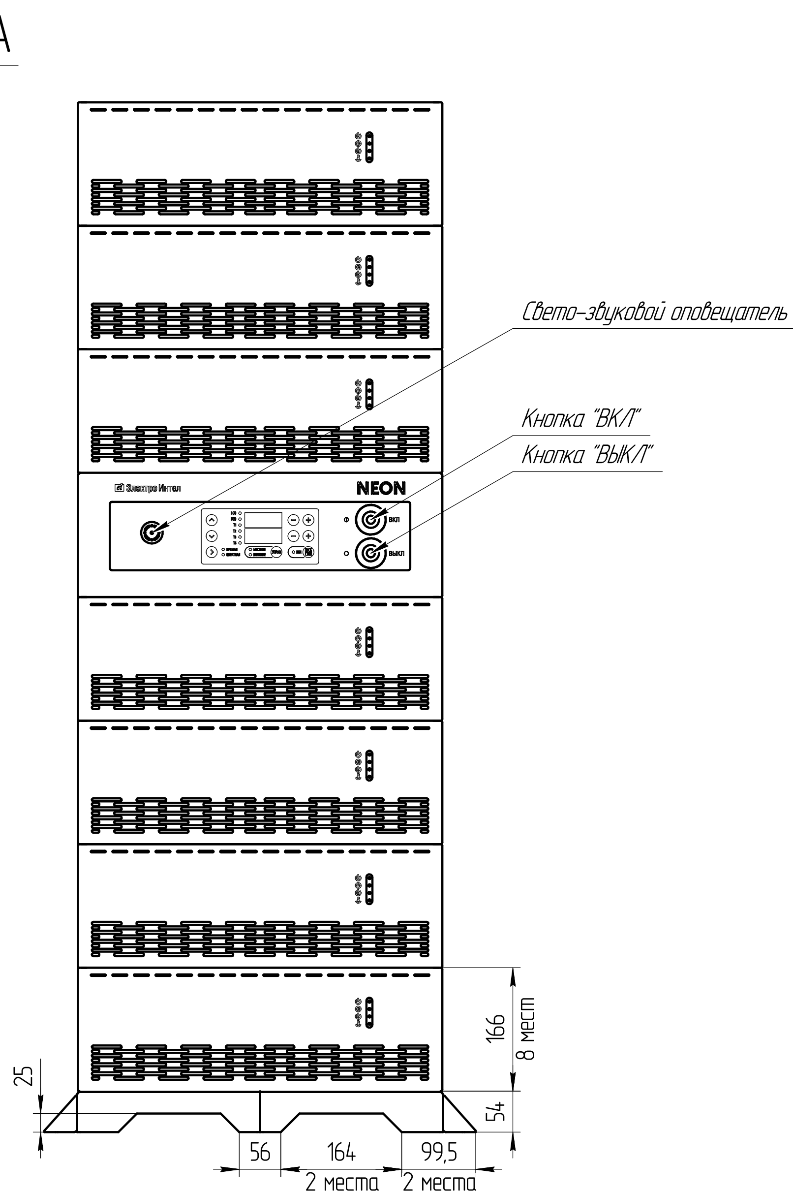
Вид спереди
