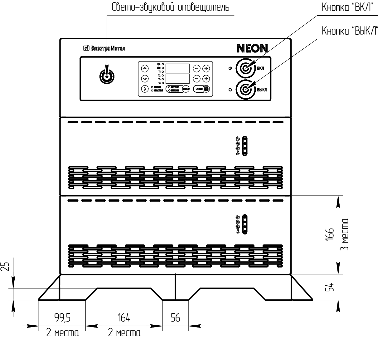
Вид спереди
