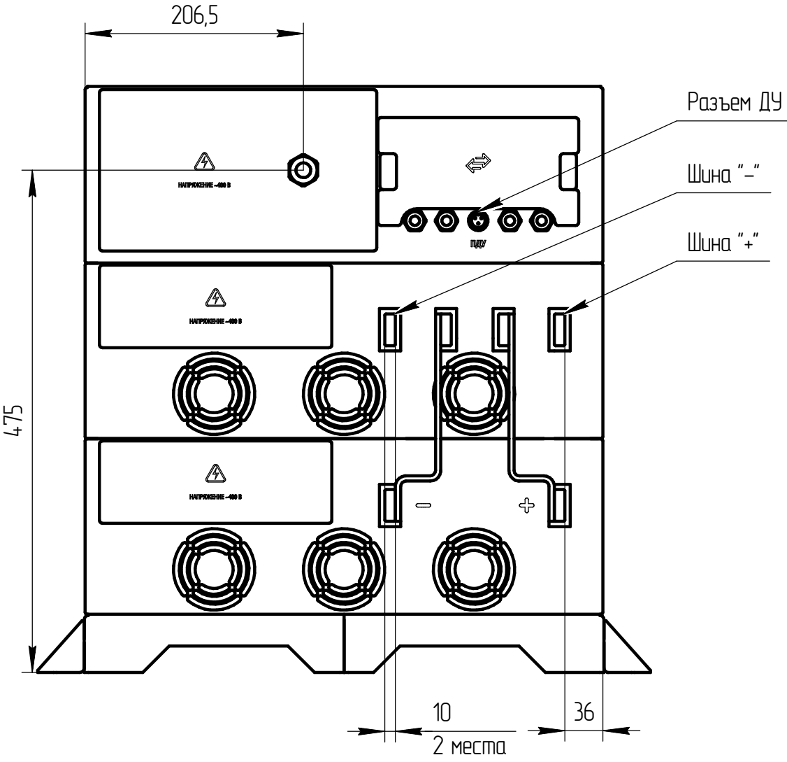
Вид сзади
