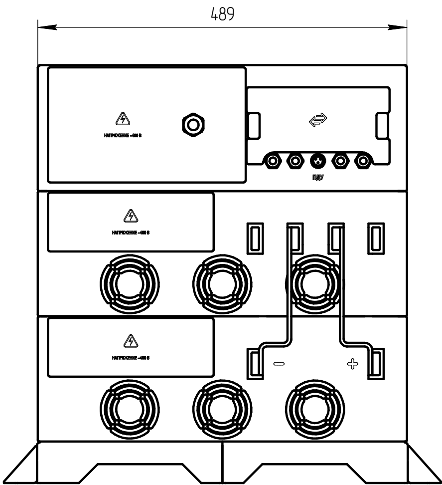
Вид сзади
