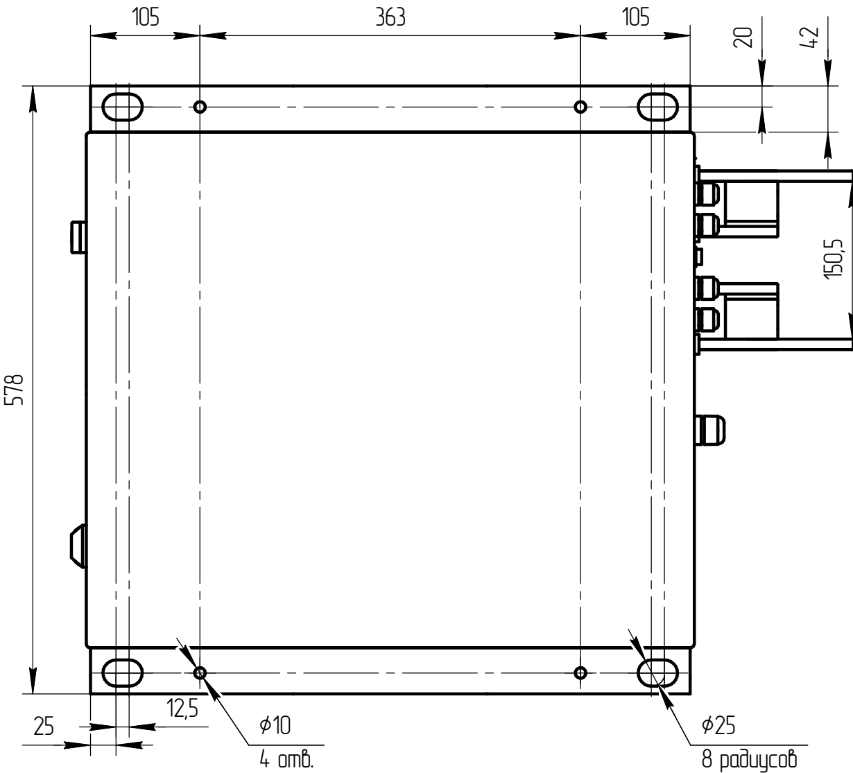
Вид сверху
