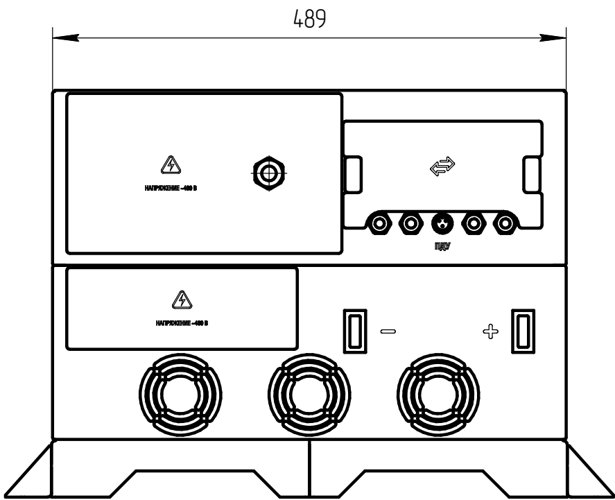
Вид сзади
