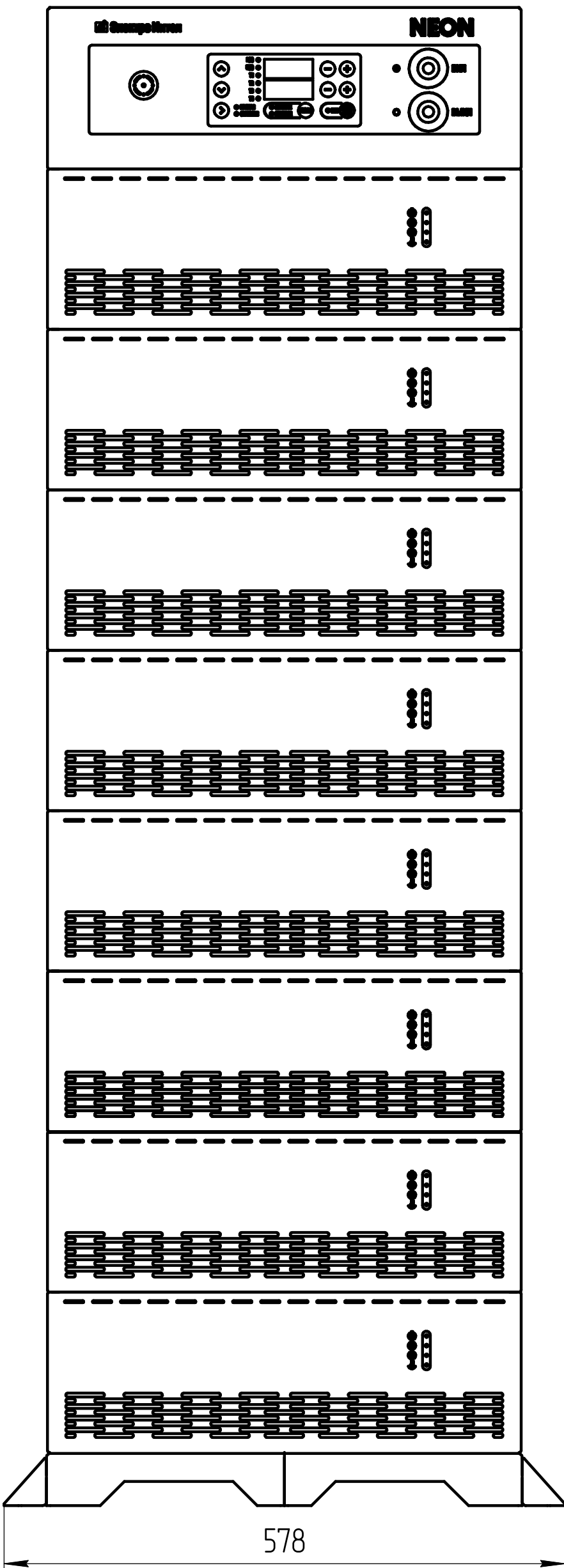
Вид спереди
