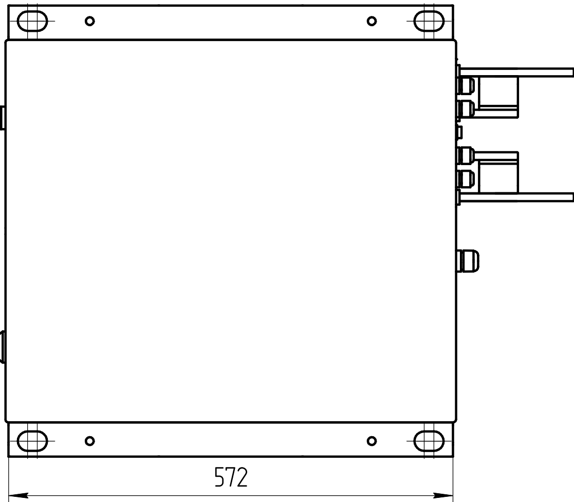
Вид сверху
