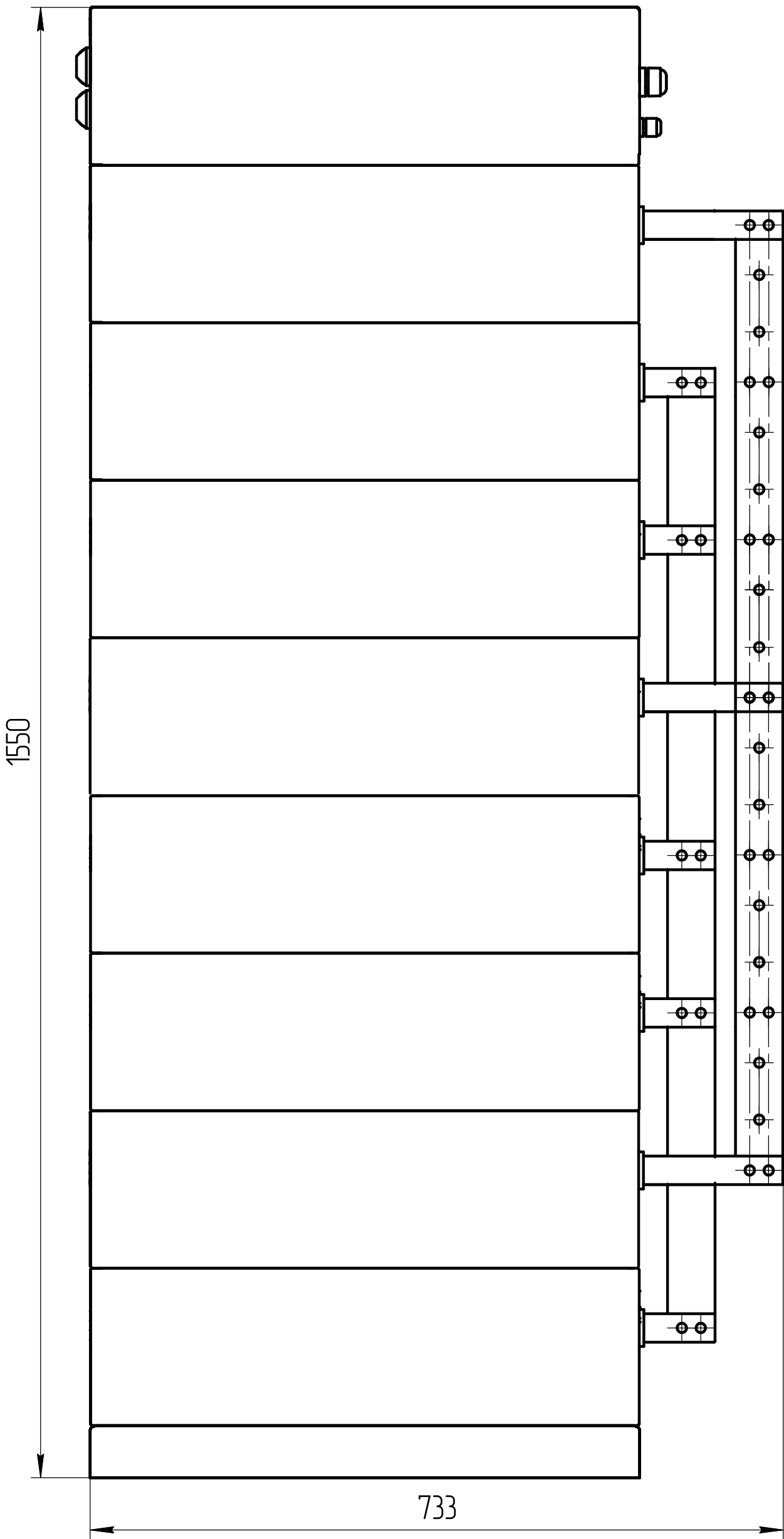
Вид сбоку
