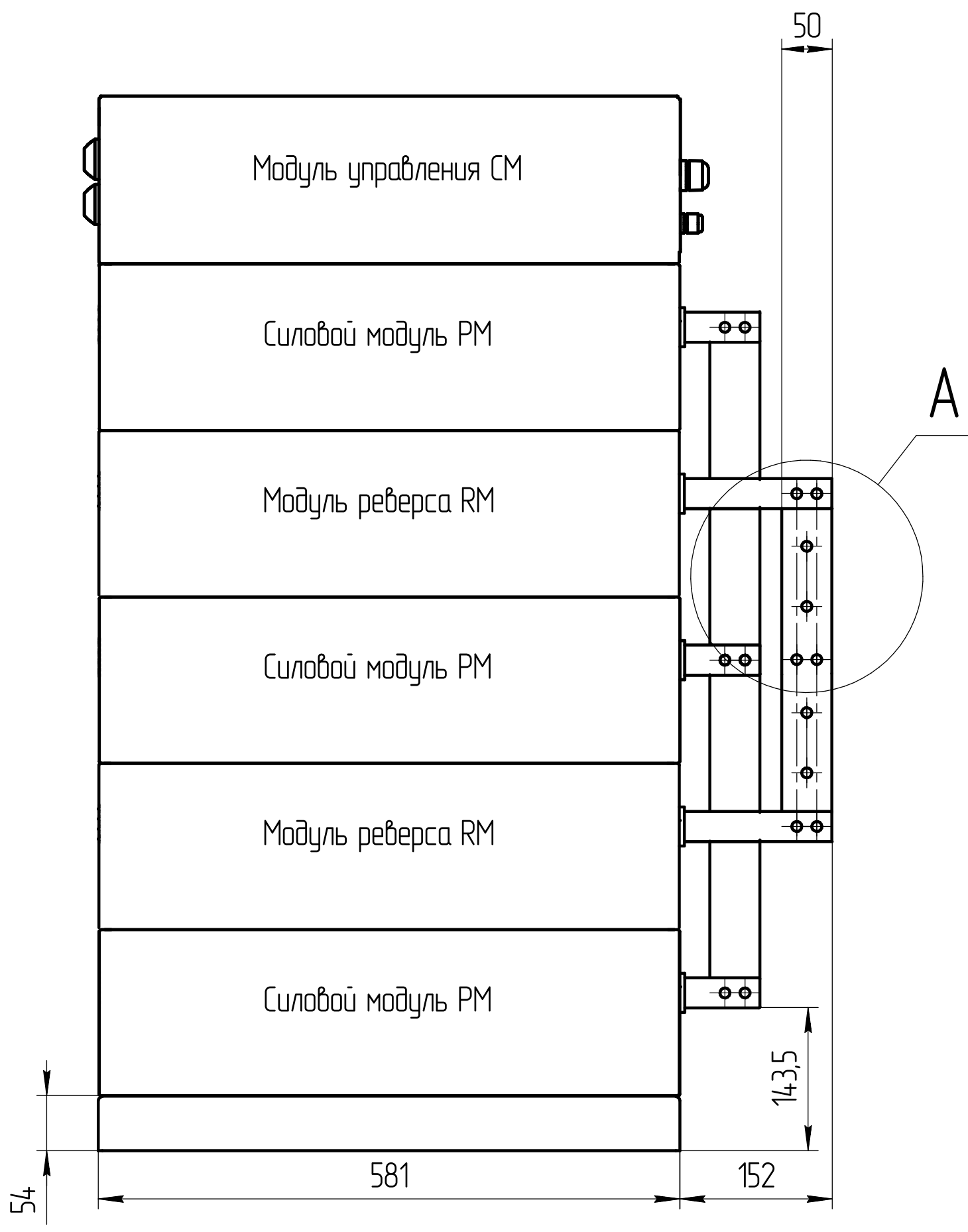
Вид сбоку
