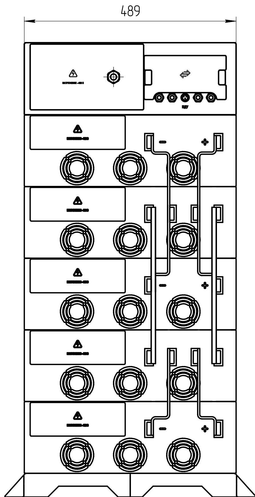
Вид сзади
