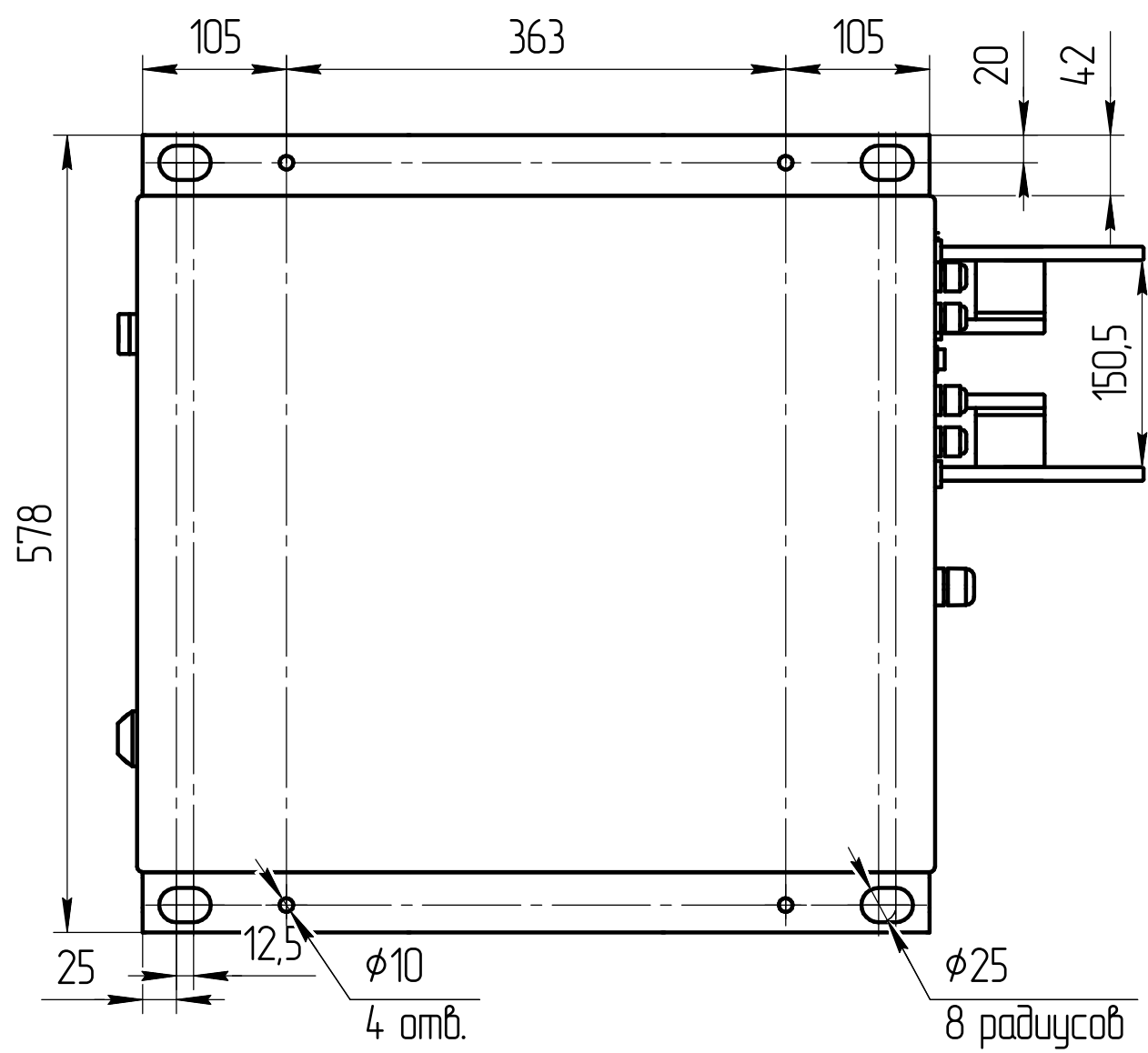
Вид сверху
