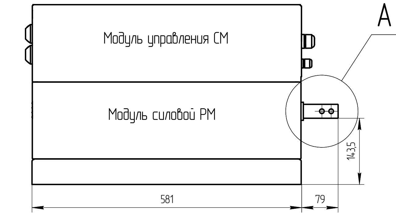
Вид сверху
