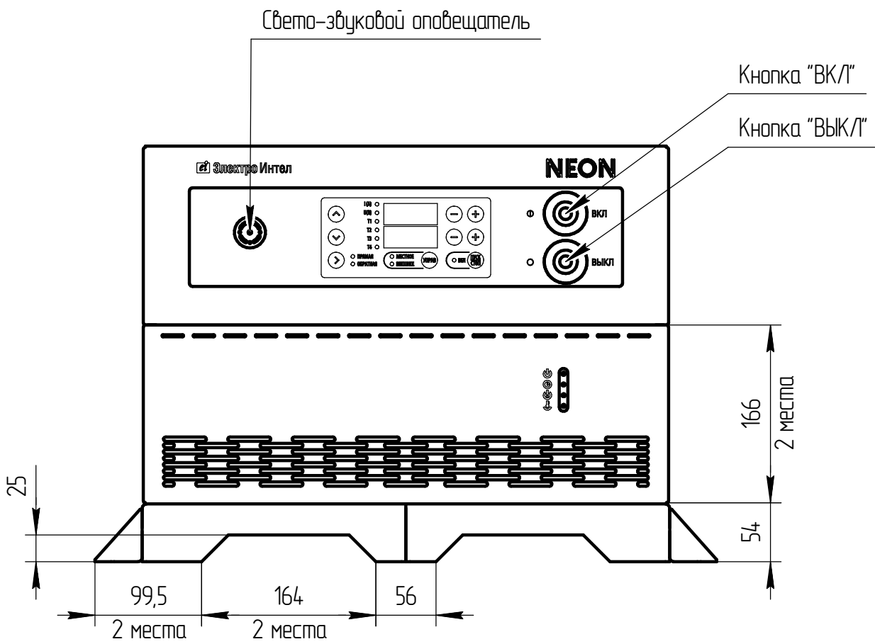
Вид спереди
