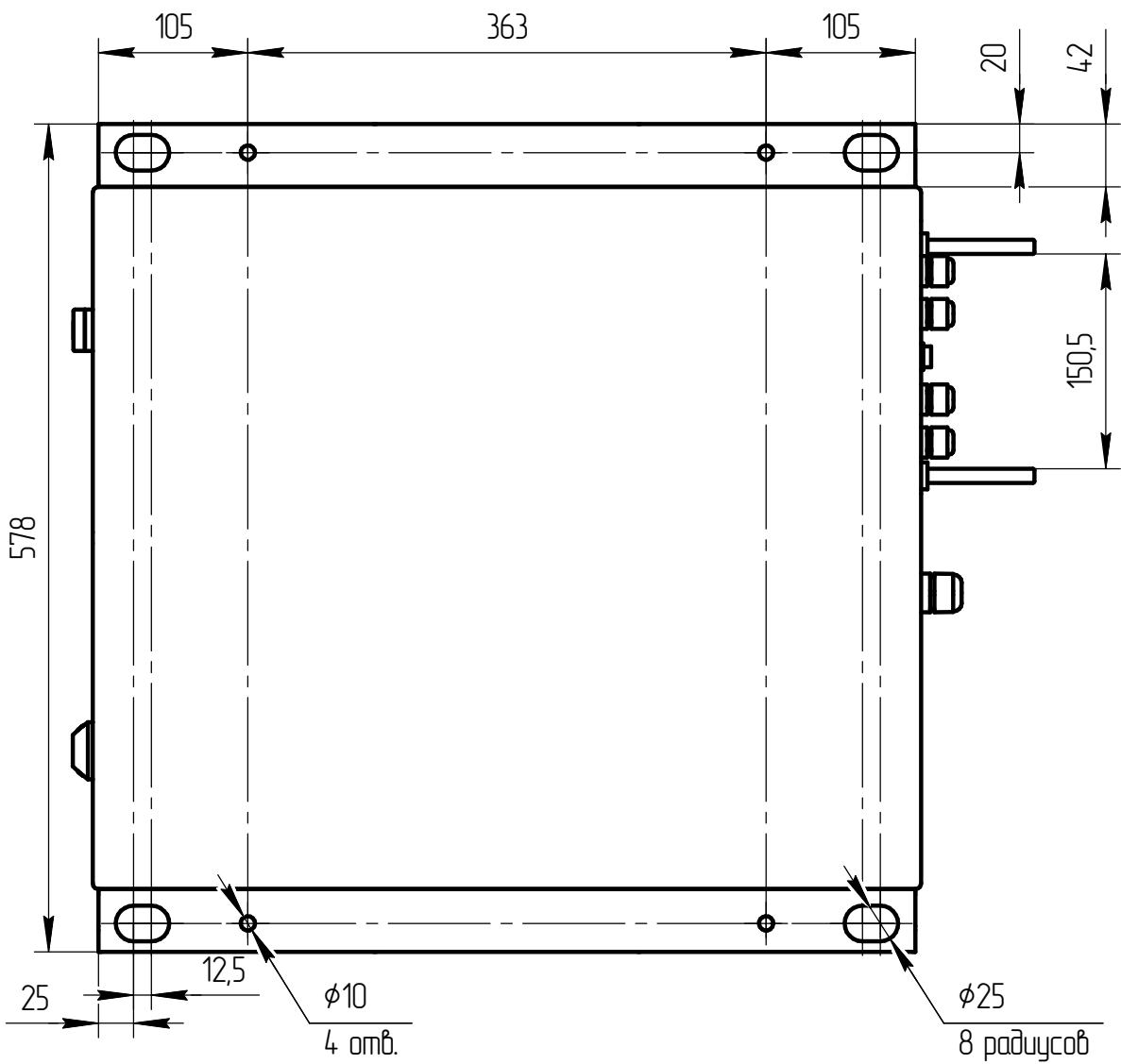
Вид сверху
