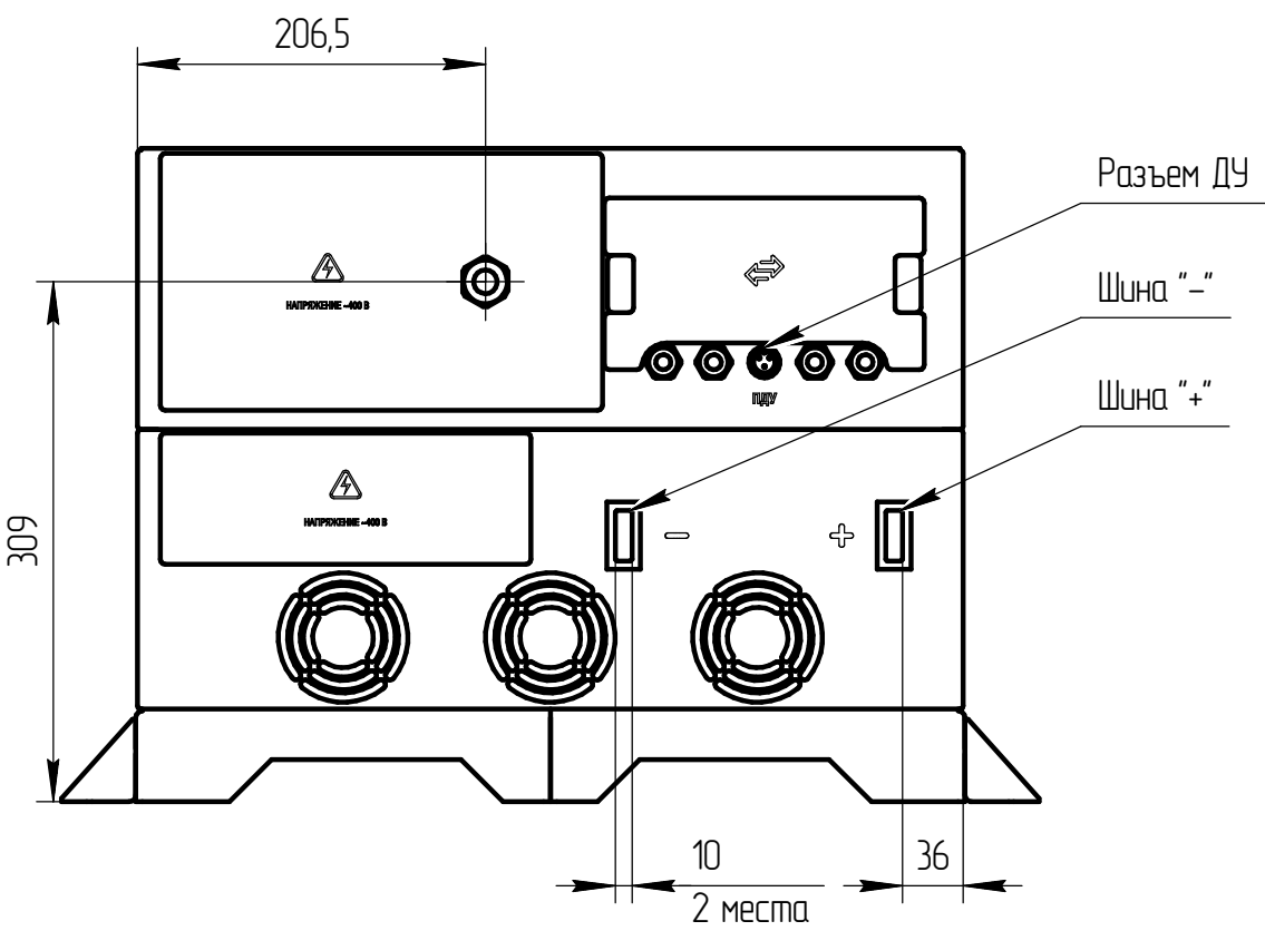
Вид сзади
