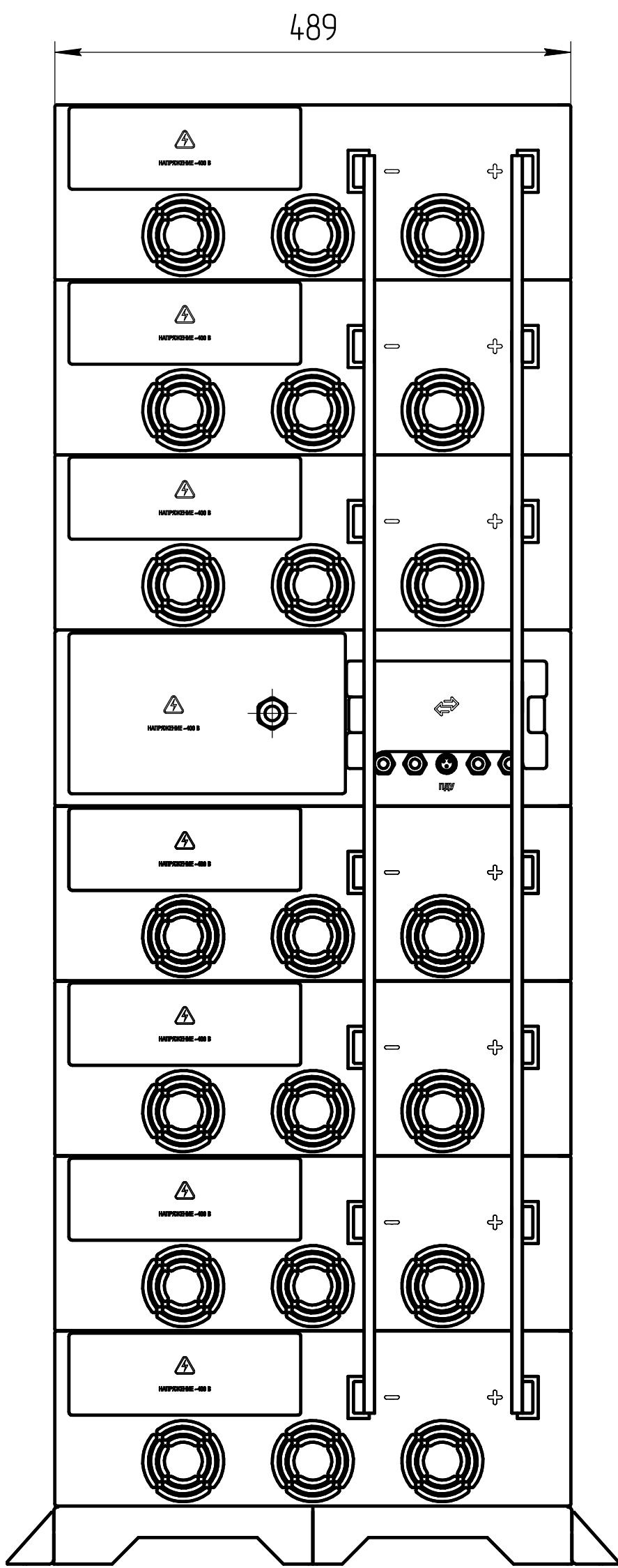
Вид сзади
