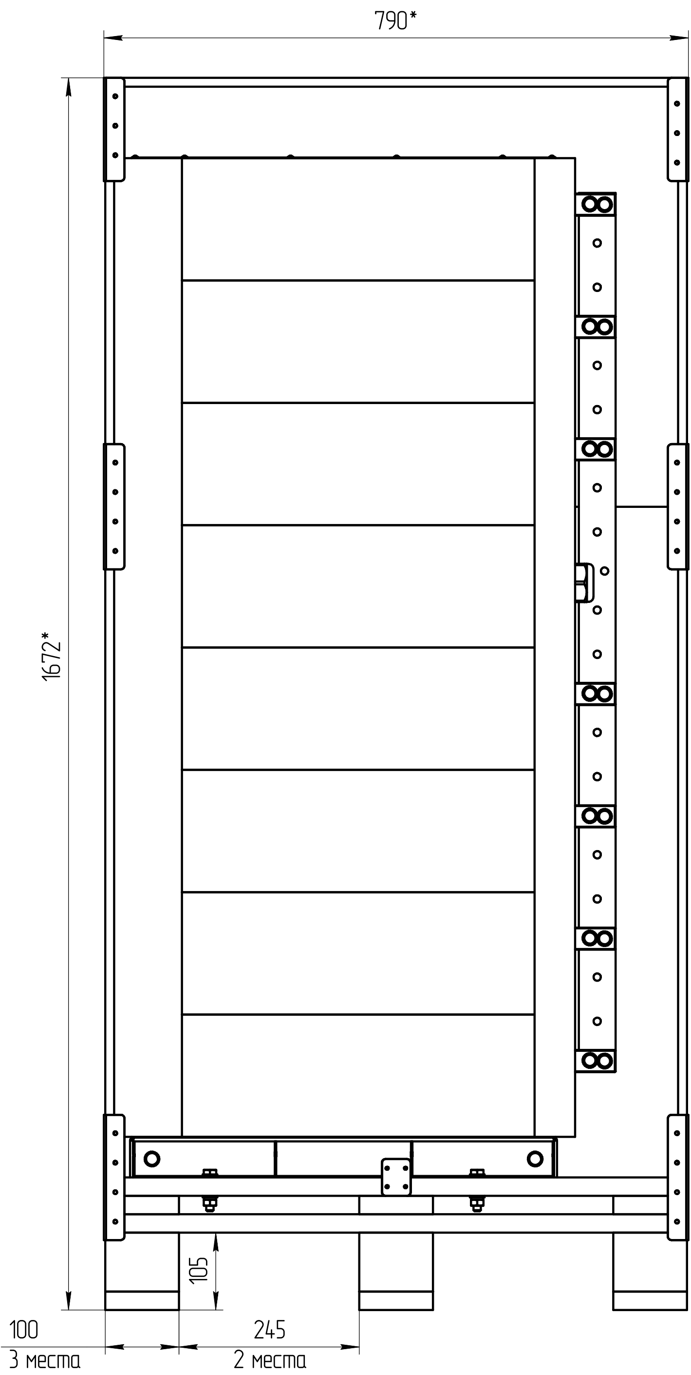
Вид сбоку
