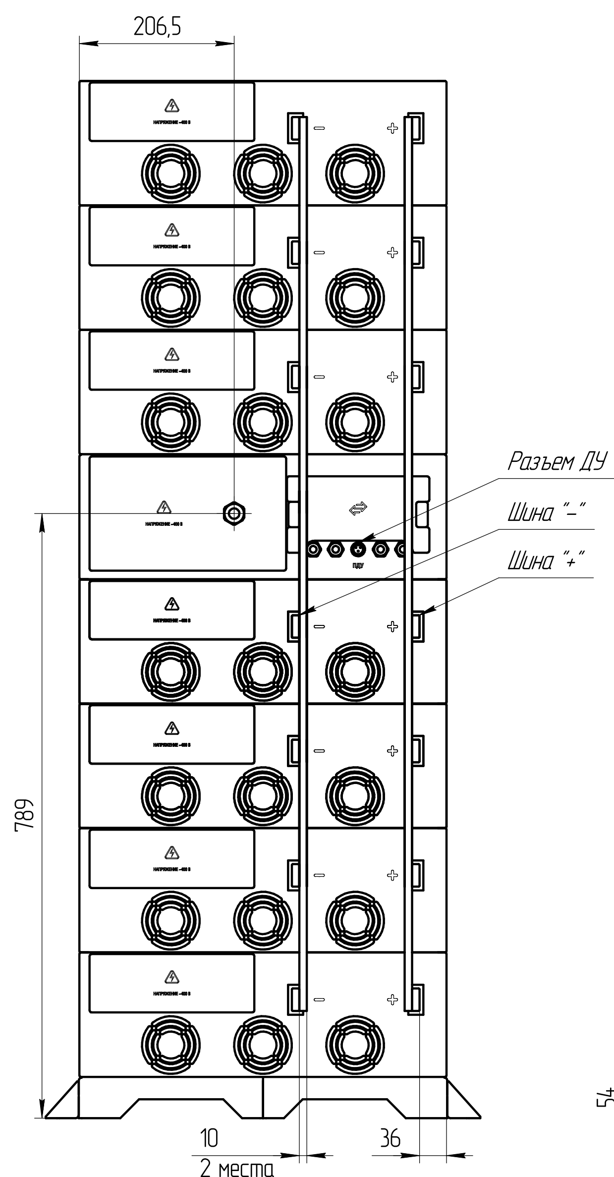
Вид сзаву
