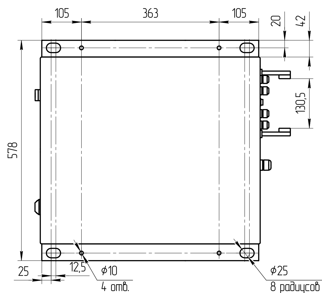
Вид сверху
