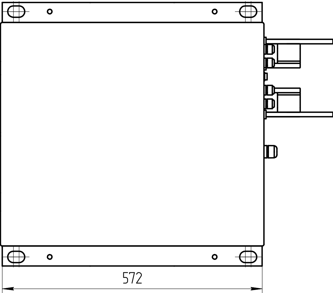
Вид сверху
