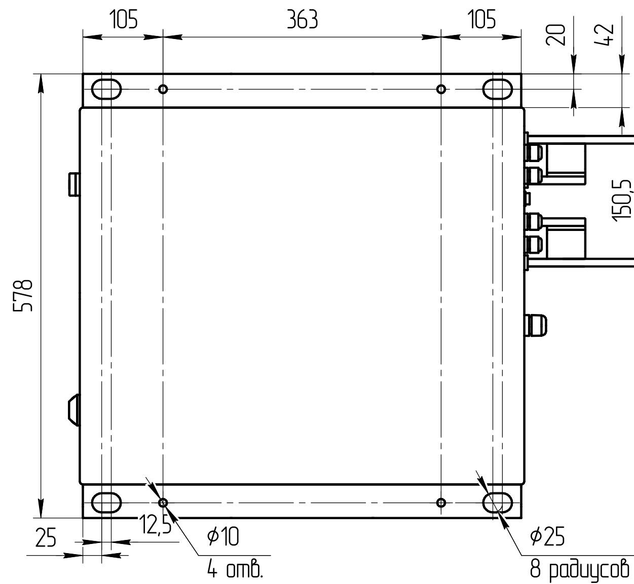
Вид сверху
