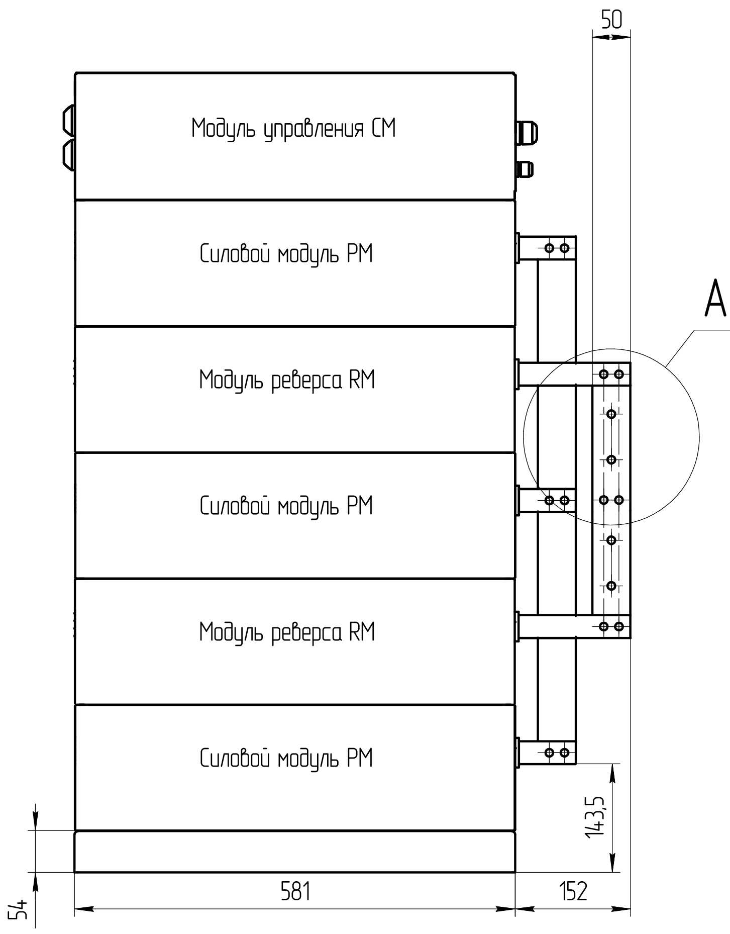
Вид сбоку
