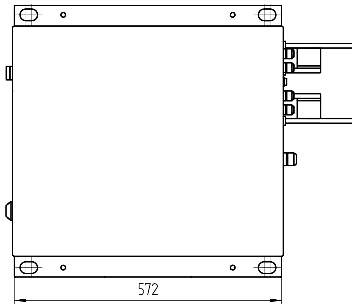
Вид сверху
