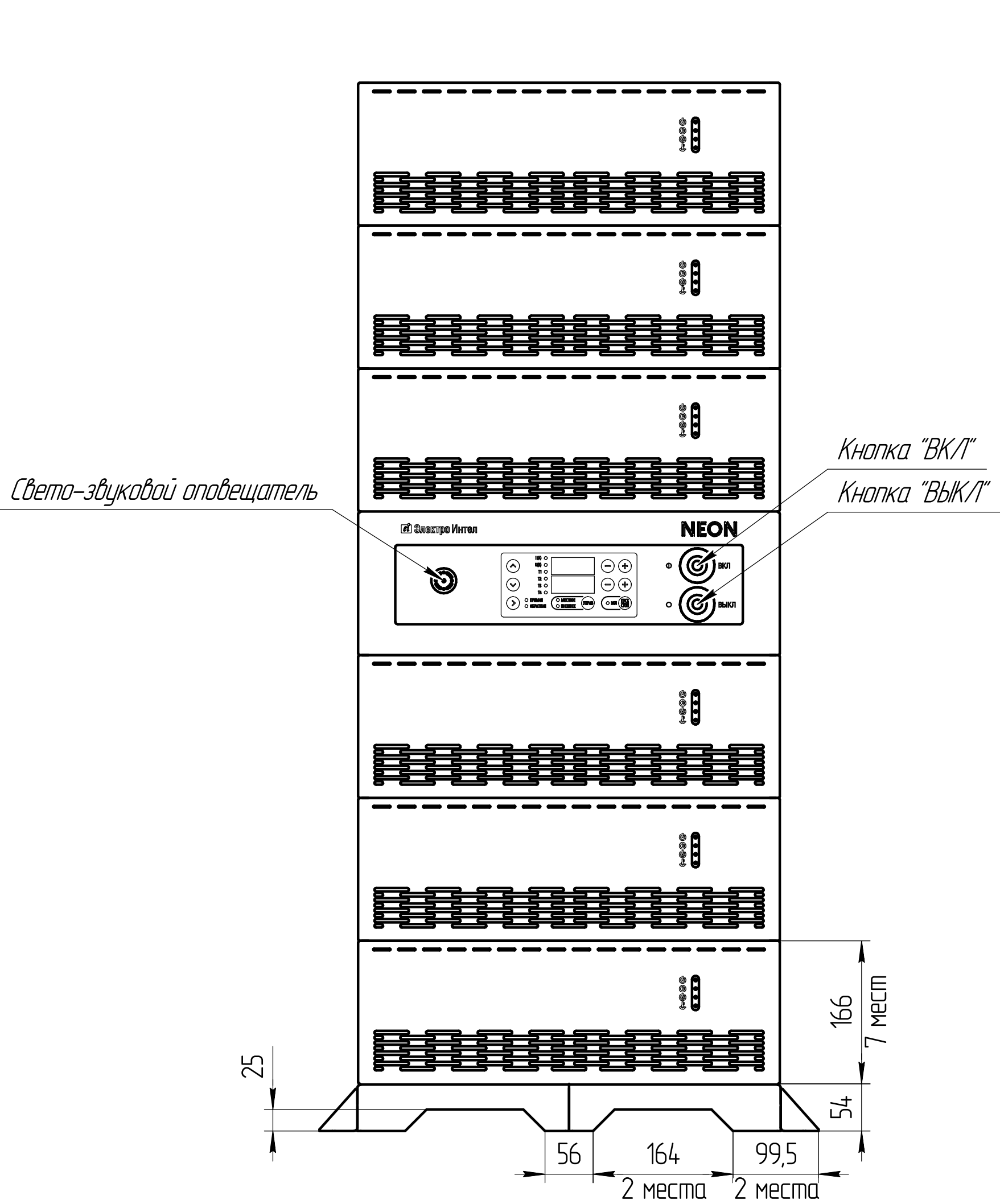
Вид спереди
