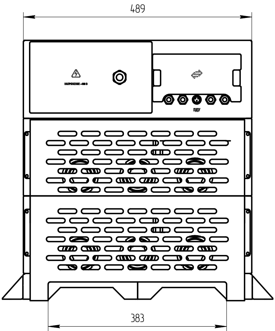
Вид сверху
