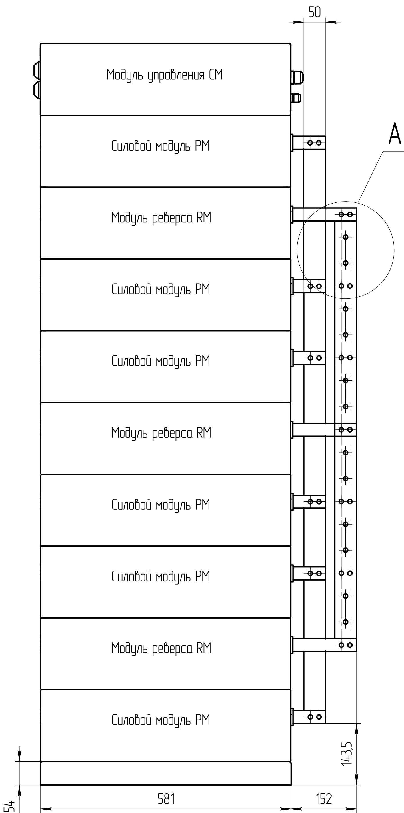
Вид сбоку
