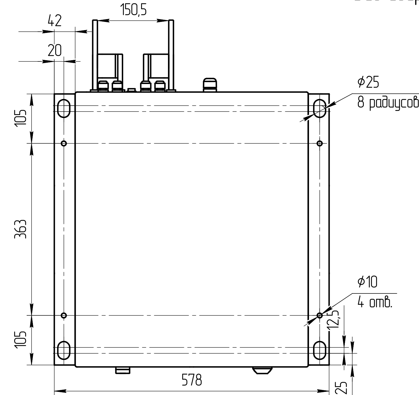
Вид сверху
