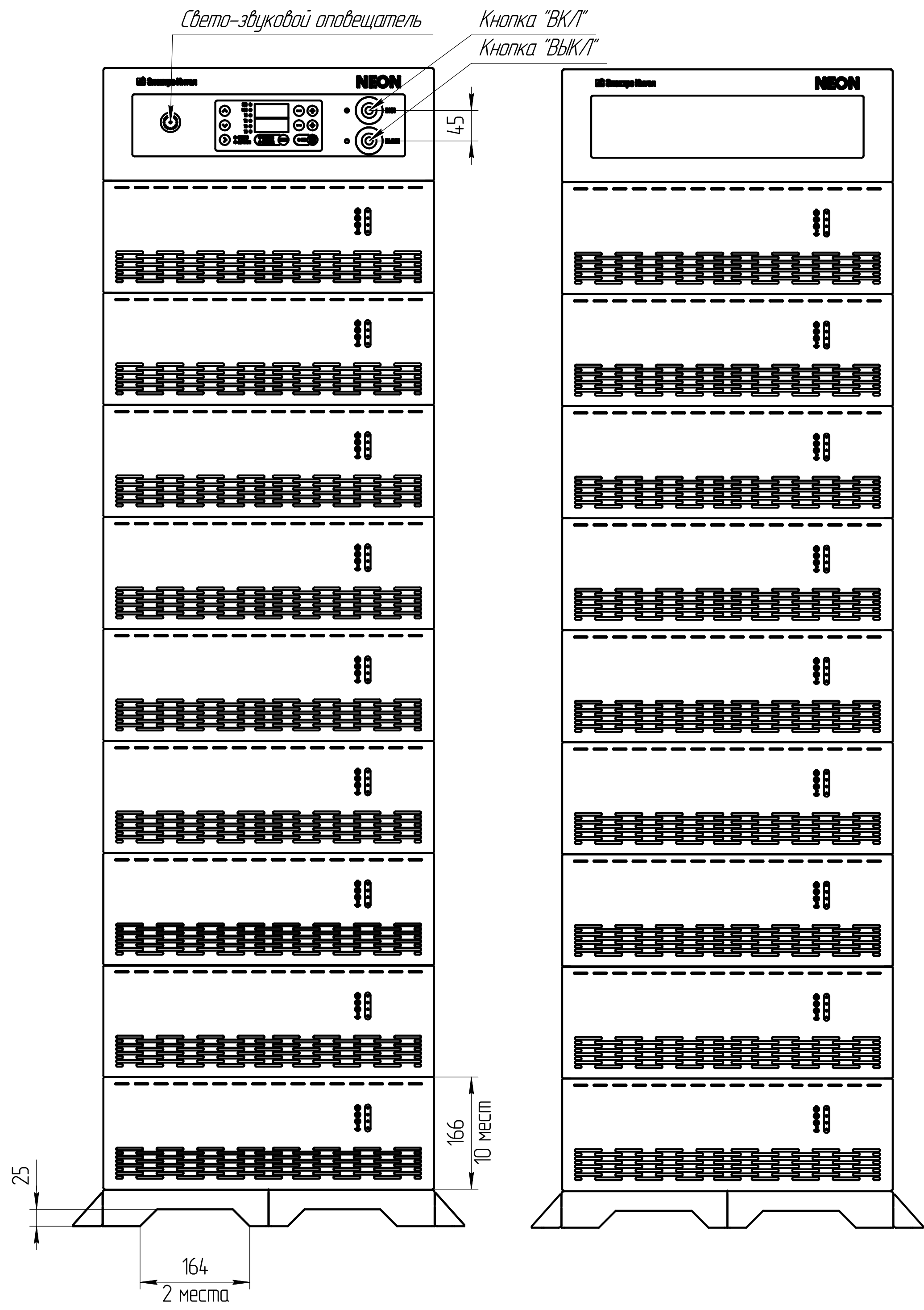
Вид спереди
